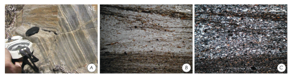
Figura 7 – Fabrica planar Sn1 [So/S1]. A) – Aspecto de Sn1 en una exposición del CEG en bajo a medio grado metamórfico. B) – Lámina delgada de la equidistancia Sn1 realizada a lo largo de la línea de estratificación, mostrando una foliación oblicua a la foliación principal, indicando cinemática del techo para el SE. C) – Misma lámina que B) pero con las polarizaciones cruzadas, mostrando la mineralogía típica con cuarzo, moscovita, biotita, clorita, cloritoides y opacos. La clorita y el cloritoides son posteriores al pico metamórfico que ha producido la asociación mineralógica de facies de la biotita, mostrando retrogradación de la misma durante el período de enfriamiento de los granitos tardívarcos (sin-3 fase) (Ferreira da Silva, 1994).
