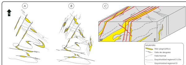
Figura 4 – Modelo esquemático para la geometría final del campo "litónico" de La Fregeneda. A) – Instalación de intrusiones pegmatíticas a lo largo de las principales discontinuidades existentes como la Sn1 (So/S1 o S2), lo S3 (Sn2), folias y fracturas de dirección N-S, NW-SE y WNW-ESE. B) – Cizallas frías (aquí representadas como dextrás) que reactivan las estructuras precoces con tectónica frágil de graben y post (WNW-ESE) generando el alineamiento de las intrusiones con el pódion observable cartográficamente. C) Bloque diagrama interpretativo de las estructuras observadas en planta y corte, con la representación de algunas fallas sinistralas. Es una representación simplificada de las geometrías observadas en el enjambre de diques pegmatíticos. Localmente se pueden superponer varias de las relaciones entre fallas representadas.
