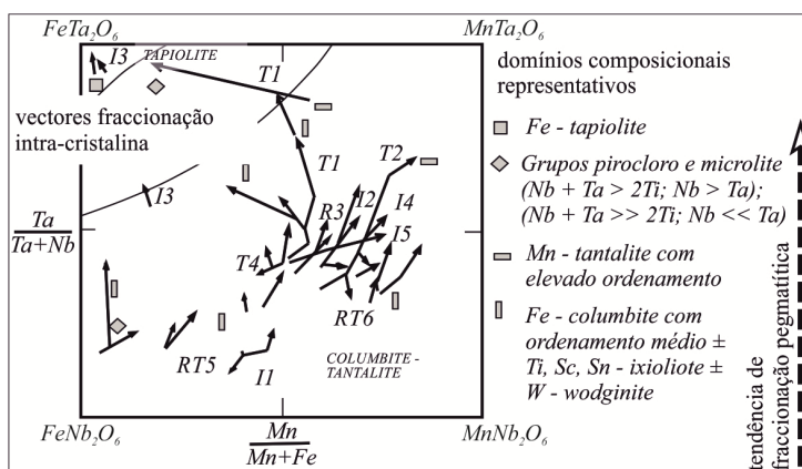
Fig. 3. Composições de minerais portadores de Nb-Ta representadas no quadrilátero da columbite-tantalite, destacando tendências de fraccionação intra-cristalina e intrapegmatíticas. Composições obtidas por análise em microsonda electrónica de cristais individualizados. Valores em apfu. Para a representação das microlites, pirocloros e ixiolites só foram ponderados os teores de Nb, Ta, Mn e Fe.
