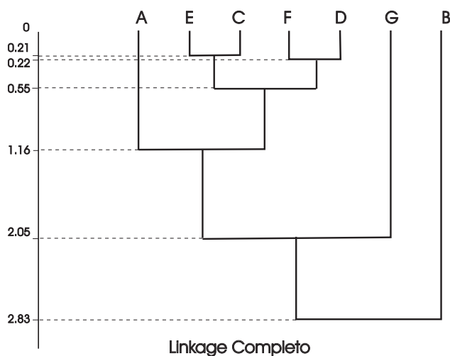
Figura 8.3: Método del amalgamamiento completo
