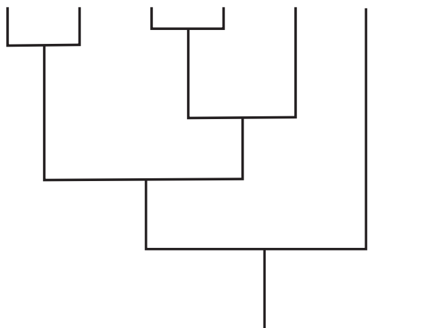
Figura 8.1: Dendrograma
