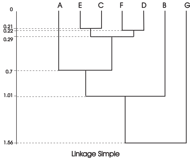
Figura 8.2: Método del amalgamamiento simple
