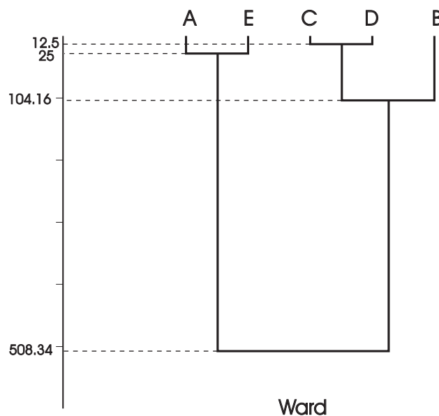
Figura 8.8: Método de Ward
