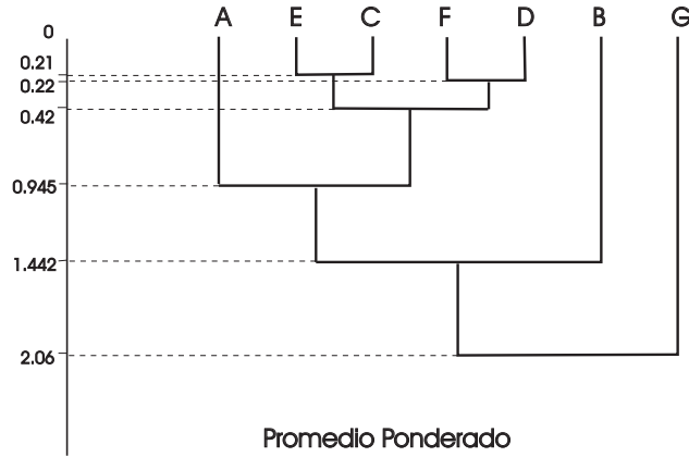
Figura 8.5: Método del promedio ponderado
