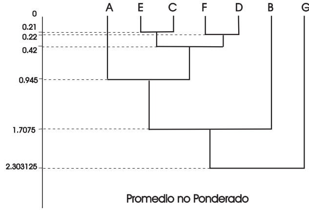
Figura 8.4: Método del promedio no ponderado
