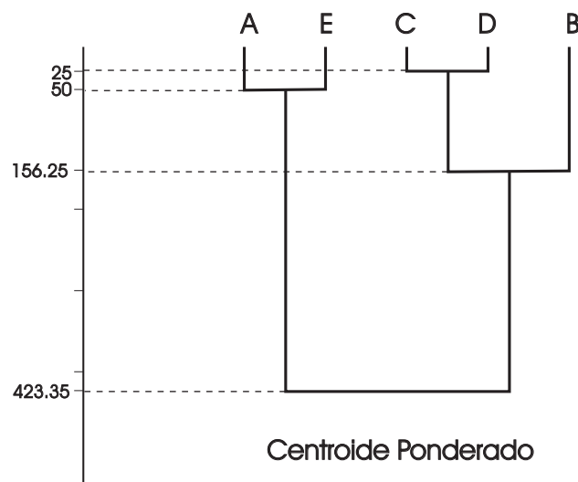
Figura 8.6: Método del centroide ponderado
