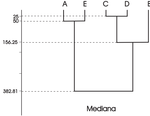
Figura 8.7: Método de la mediana
