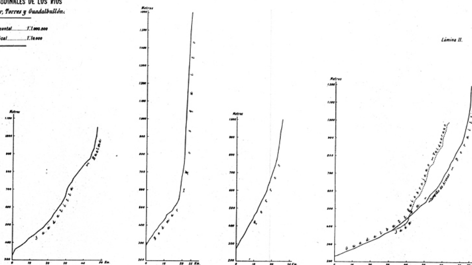
PERFILES LONGITUDINALES DE LOS RÍOS Jandulilla, Bedmar, Torres y Guadalbullón.
