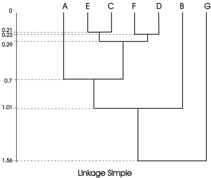
Dendrograma
