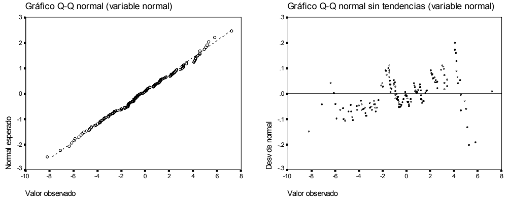
Figura 11.11.a. Gráficos de normalidad: muestra extraída de una distribución normal .
