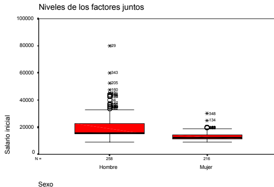
Figura 11.5.a. Diagramas de caja de la variable salini (salario inicial) en hombres y mujeres .
