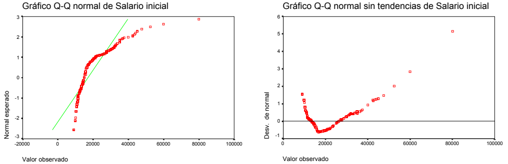
Figura 11.10. Gráficos de normalidad del procedimiento Explorar .
