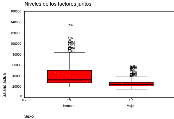
Figura 11.5.b. Diagrama de caja de la variable salario (salario actual) en hombres y mujeres .
