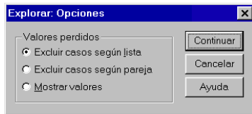
Figura 11.13. Subcuadro de diálogo Explorar: Opciones .
