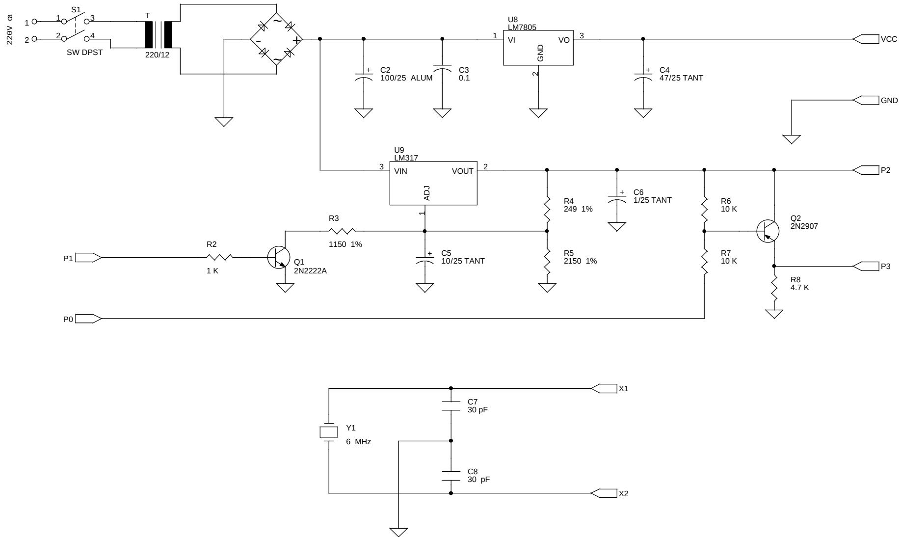
Esquema de la Fuente de Alimentación
