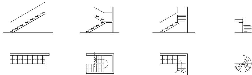
Escalera de un tramo recto Escalera en U o de dos tramos Escalera en L con descansillo Escalera de caracol
