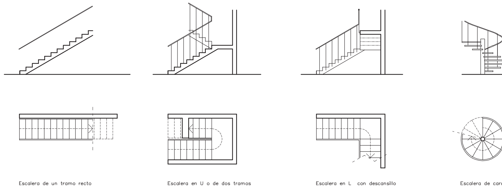
Escalera de un tramo recto
