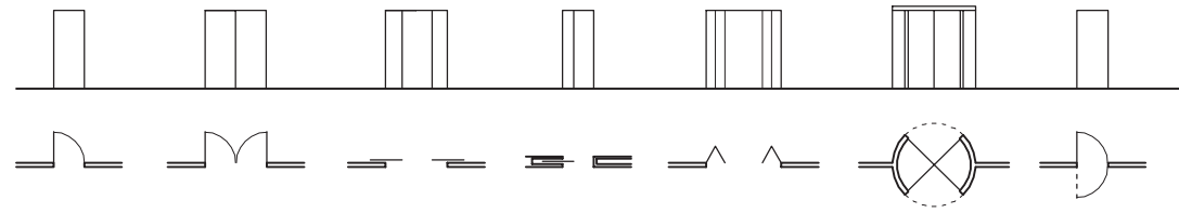
Puerta abatible Puerta doble Puerta corredera Puerta corredera Puerta plegable Puerta giratoria Puerta de vaivén
