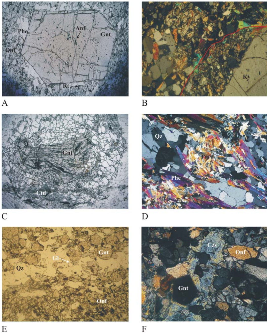
FIGURA 2. Microfotografías de las rocas de alta presión de la Península de La Guajira. Eclogitas: A. Porfiroblasto idiomórfico de granate zonado en la matriz. Se aprecian las inclusiones de anfíbol verde. B. En el borde derecho se observa un porfiroblasto de cianita, con dos generaciones de crecimiento. La línea roja demarca el límite del cristal poikilítico. Esquistos: C. Porfiroblasto xenomórfico de granate con dos generaciones de crecimiento. D. Cianita retrogradada a mica blanca (par?). Gneises: E. Bandeamiento definido por variaciones en tamaño de grano y composición. F. Crecimiento de clinozoisita a partir de cuarzo, onfacita y glaucofana. Abreviaturas: Anf – anfíbol, Ctd – cloritoide, Czs – clinozoisita, Gl – glaucofana, Gnt – granate, Ky – cianita, Onf – onfacita, Par – paragonito, Phe – fengita, Qz – cuarzo, Rt – rutilo.
