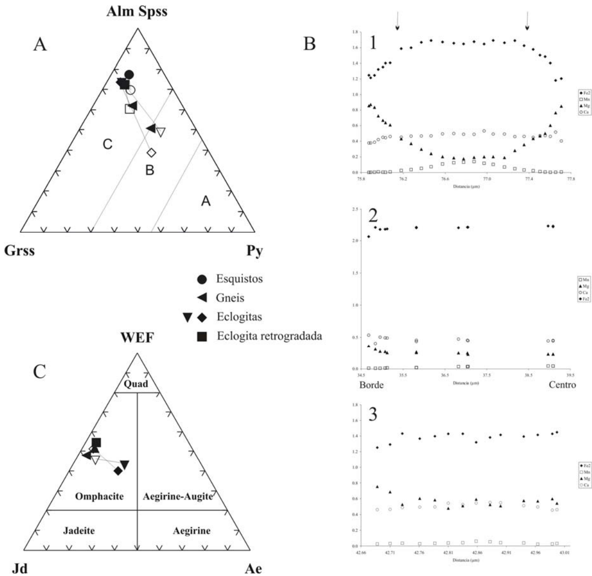
FIGURA 3. Química mineral. A. Clasificación de granates. Los símbolos sin relleno representan las composiciones de los bordes. Las líneas unen centros y bordes para los minerales. B. Perfiles de zonación para granates representativos de La Guajira. 1. Eclogitas, 2. Esquitos, 3. Gneises. C. Clasificación de piroxenos. Los símbolos sin relleno representan las composiciones de los bordes. Las líneas unen centros y bordes para los minerales.
