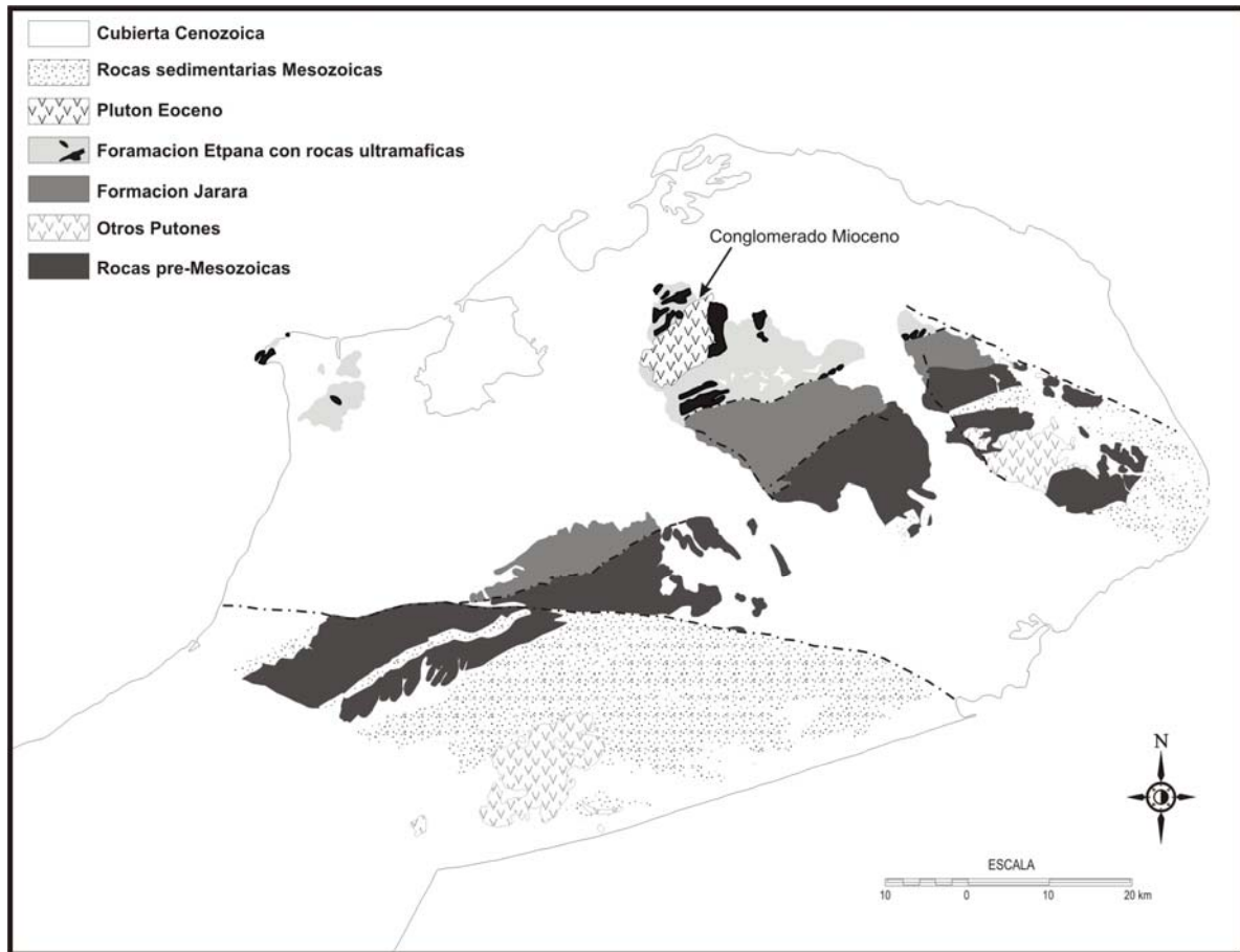
FIGURA 1. Mapa geológico generalizado de la Península de La Guajira, Colombia. La flecha indica la localización del conglomerado Mioceno.
