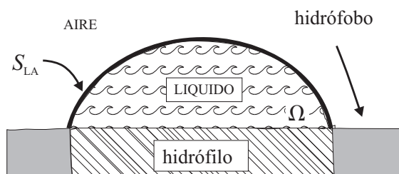
Figura 2: Una gota líquida apoyada sobre un substrato hidrófilo \Omega .
