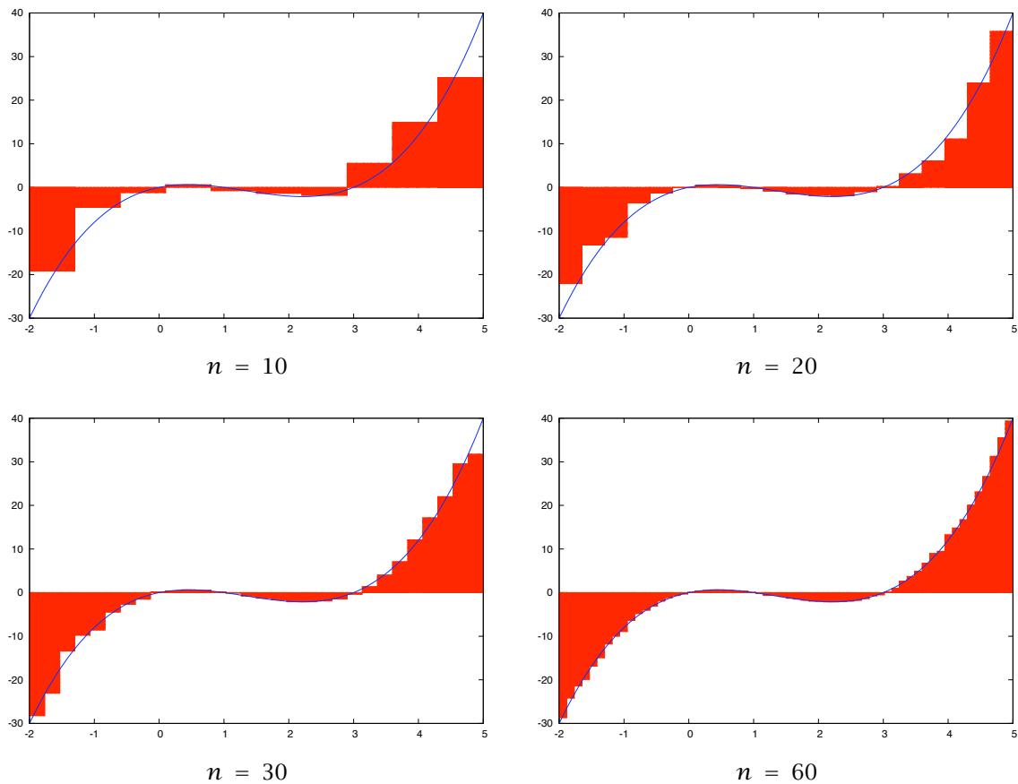
Figura 8.3 Convergencia de las sumas de Riemann
