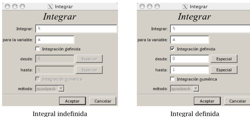
Figura 8.1 Cálculo de integrales
