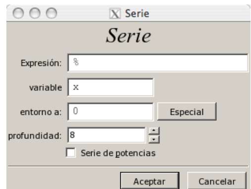
Figura 7.2 Ventana para el cálculo de la serie de Taylor
