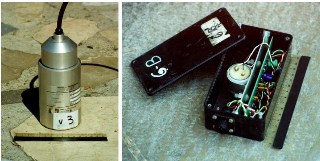
Figura 2.2. (izquierda) Sensor sísmico vertical Mark L4C. (derecha) Sensor sísmico vertical Mark L15B, junto con la electrónica de la extensión de respuesta y preamplificación.
