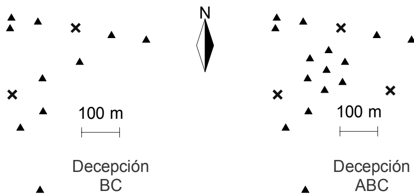
Figura 2.2. Configuración de los arrays sísmicos instalados en la isla Decepción durante las campañas 94-95 (izquierda) y 95-96 y 96-97 (derecha).
