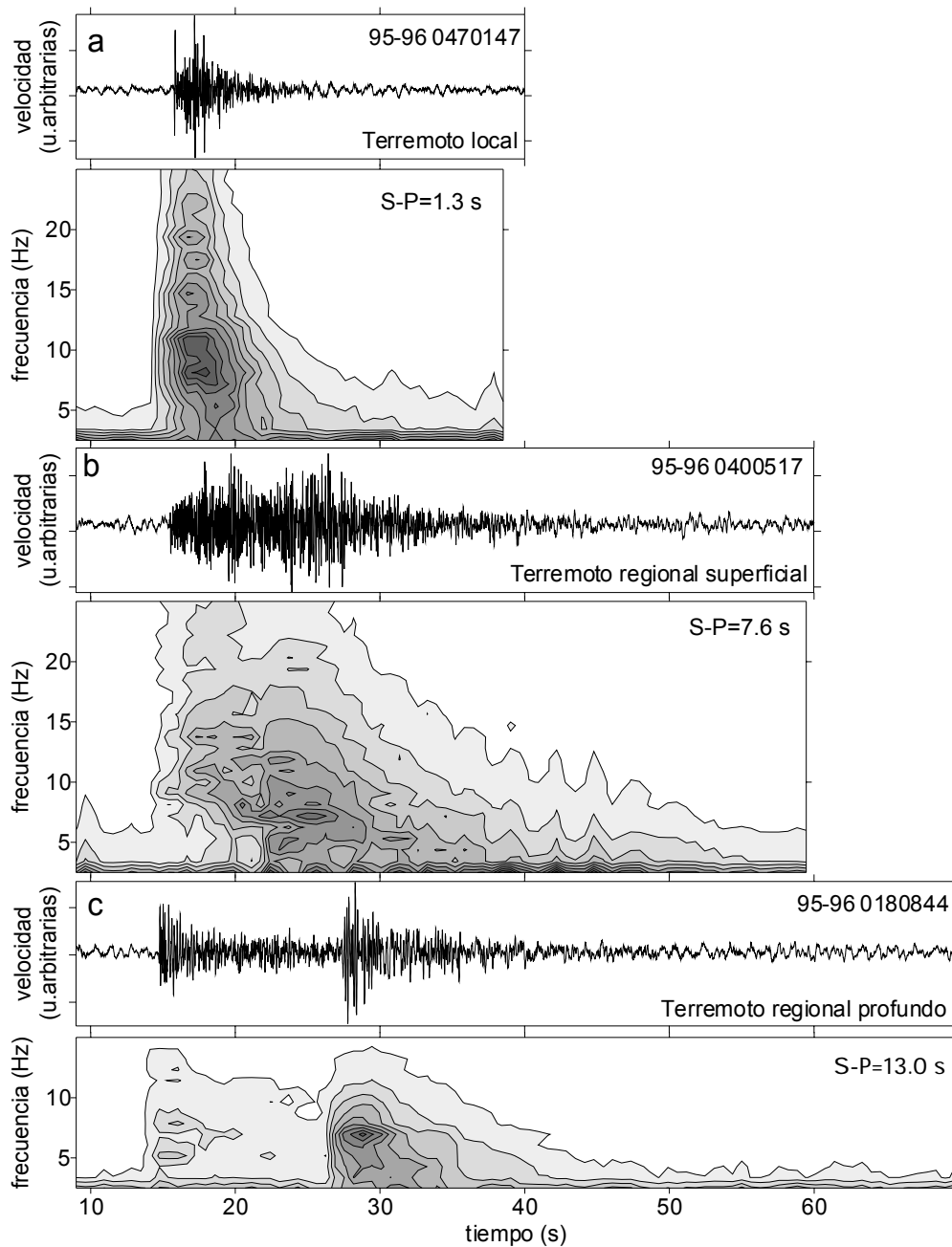
Figura 4.1. Sismogramas de componente vertical y espectrogramas promedio correspondientes para un terremoto local (a) y dos regionales (b y c). Posteriormente se demostrará que (b) es un terremoto superficial, mientras que (c) es profundo.
