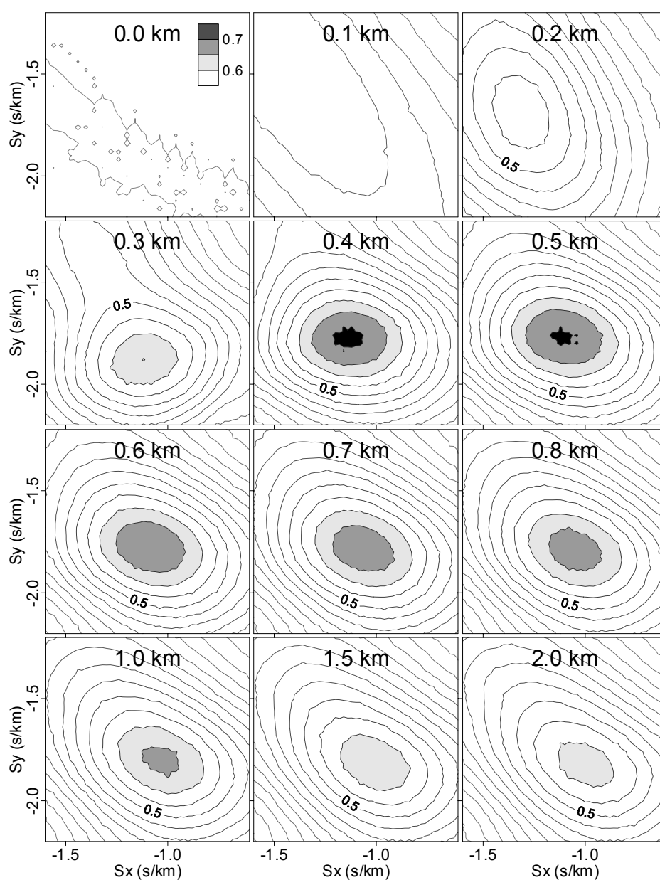
Figura 6.28. Ejemplo de contornos de CCP sobre el plano de lentitud aparente a diferentes distancias, calculado utilizando el método del frente de onda circular. Obsérvese la aparición de un máximo a una distancia de 0.4-0.5 km (de ALMENDROS ET AL., 1998).
