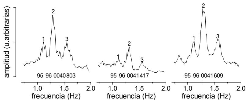
Figura 9.1. Espectro de tres registros de actividad de largo periodo.
