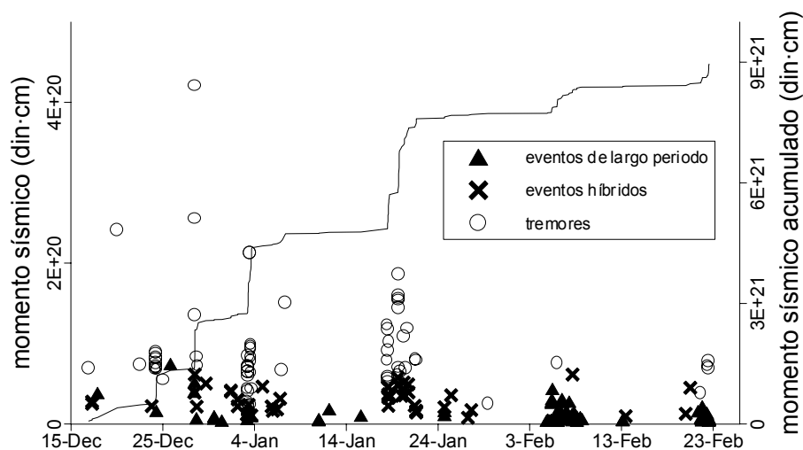
Figura 10.1. (símbolos, eje izquierdo) Momento sísmico de los eventos sismo-volcánicos pertenecientes a la campaña 95-96 que han sido localizados. (línea continua, eje derecho) Momento sísmico acumulado.
