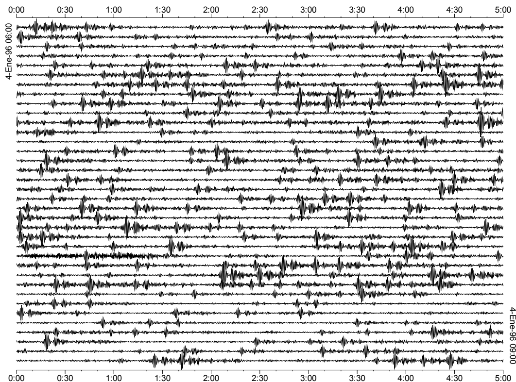
Figura 5.4. Tres horas de registro continuo durante el periodo de actividad que tuvo lugar el 4 de enero de 1995.
