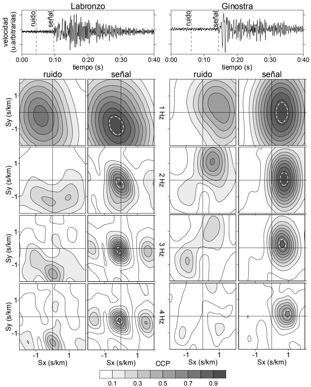
Figura 4.1. Ejemplos de localización en las distintas bandas de frecuencia utilizando el método de la CCP para una explosión registrada en los arrays de Labronzo (izquierda) y Ginostra (derecha). La primera ventana corresponde al ruido pre-evento, mientras que la segunda contiene el comienzo de la señal.
