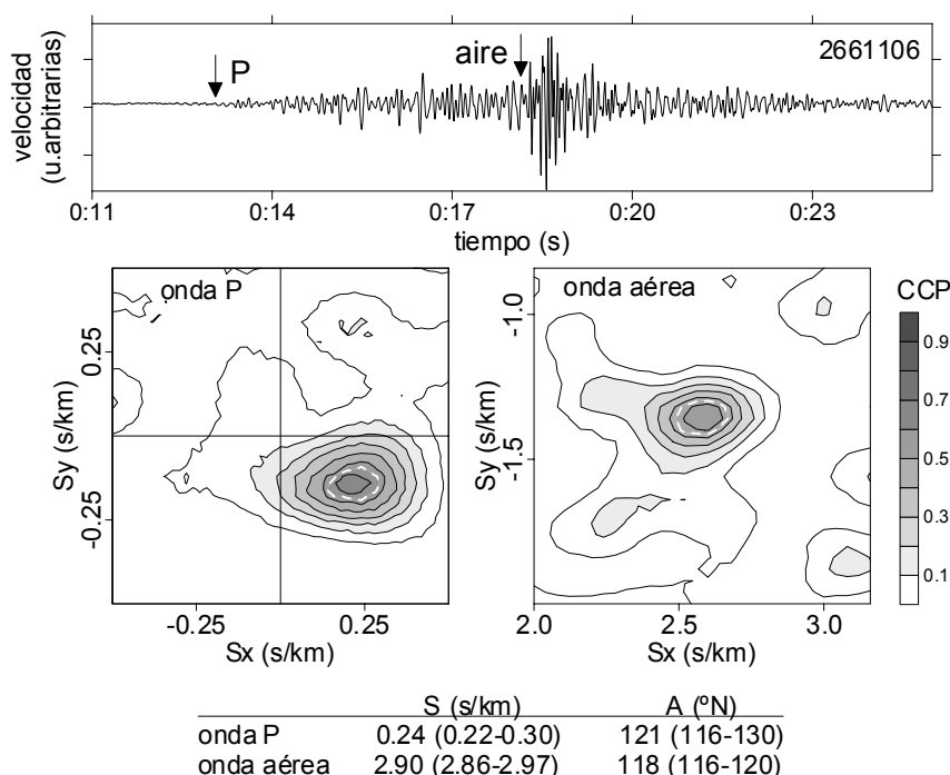
Figura 4.3. Resultados del análisis de la CCP sobre el plano de lentitud aparente para la onda P y la onda aérea de una explosión. Se muestra el apilamiento de los resultados en las bandas de frecuencia por encima de 2 Hz. El contorno discontinuo indica el intervalo de error.
