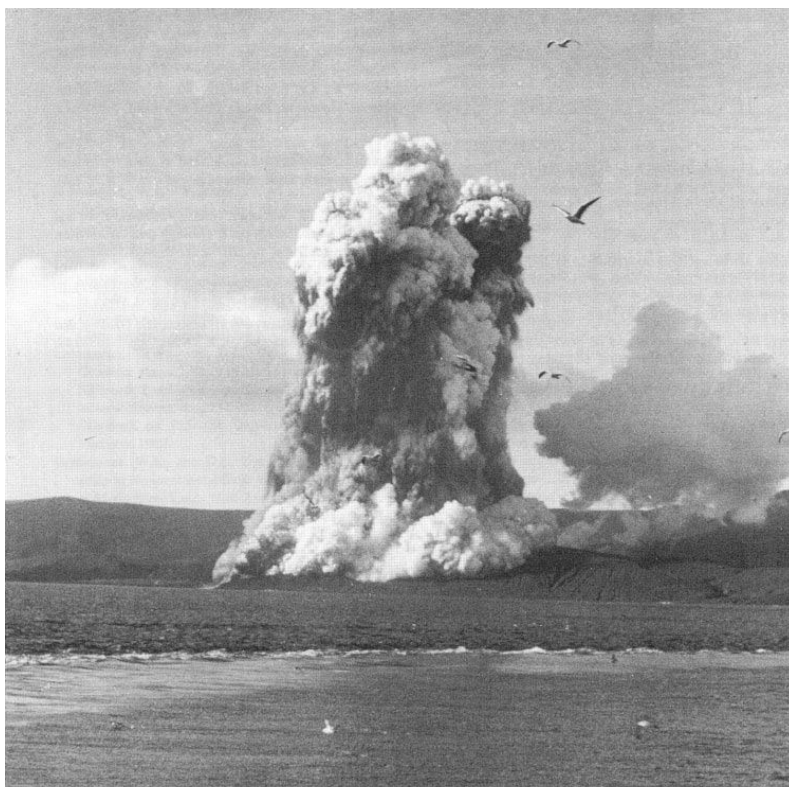
Figura 1.7. Otro momento de las erupciones de 1967 de la isla Decepción (de LEMASURIER & THOMSON, 1990)
