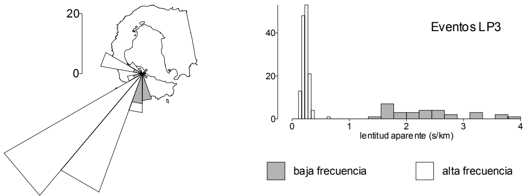
Figura 6.9. Histogramas de los resultados obtenidos para todos los eventos de largo periodo de tipo LP3.
