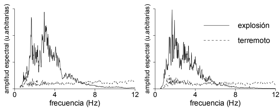
Figura 3.3. Espectros de las señales que aparecen en las Figuras 3.1 (explosión, línea continua) y 3.2 (terremoto, línea discontinua).
