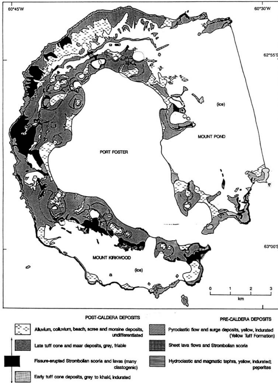
Figura 1.3. Esquema geológico de la isla Decepción (de SMELLIE ET AL., 1997)
