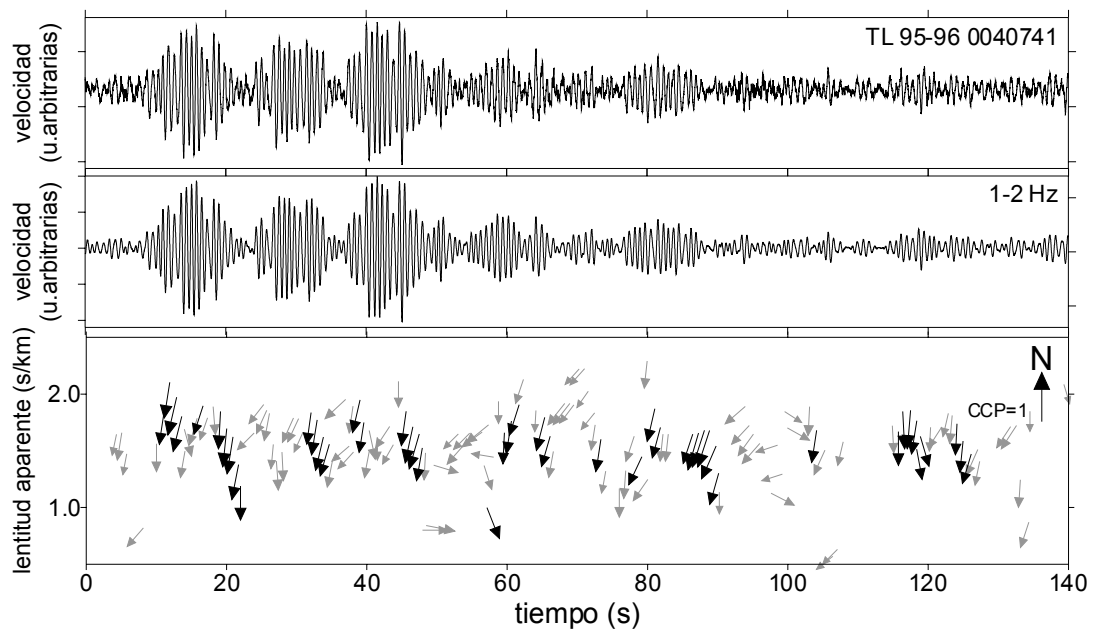
Figura 6.20. Resultados del método de la CCP a lo largo del tiempo para un episodio de trémor de baja frecuencia TL.
