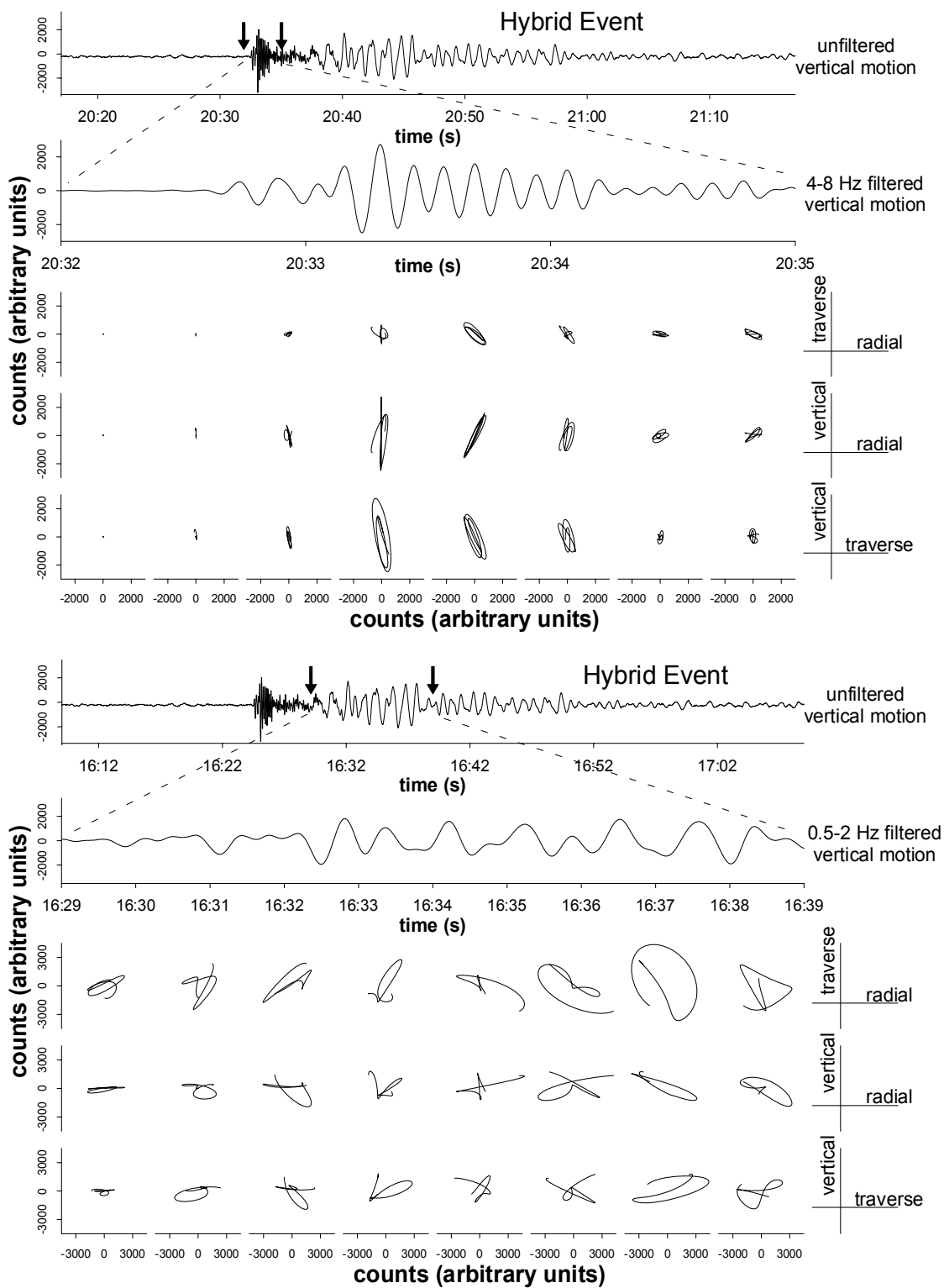
Figura 7.2. Movimiento de la partícula para las ondas de alta (arriba) y de baja frecuencia que componen los eventos híbridos (de DEL PEZZO ET AL., 1998).
