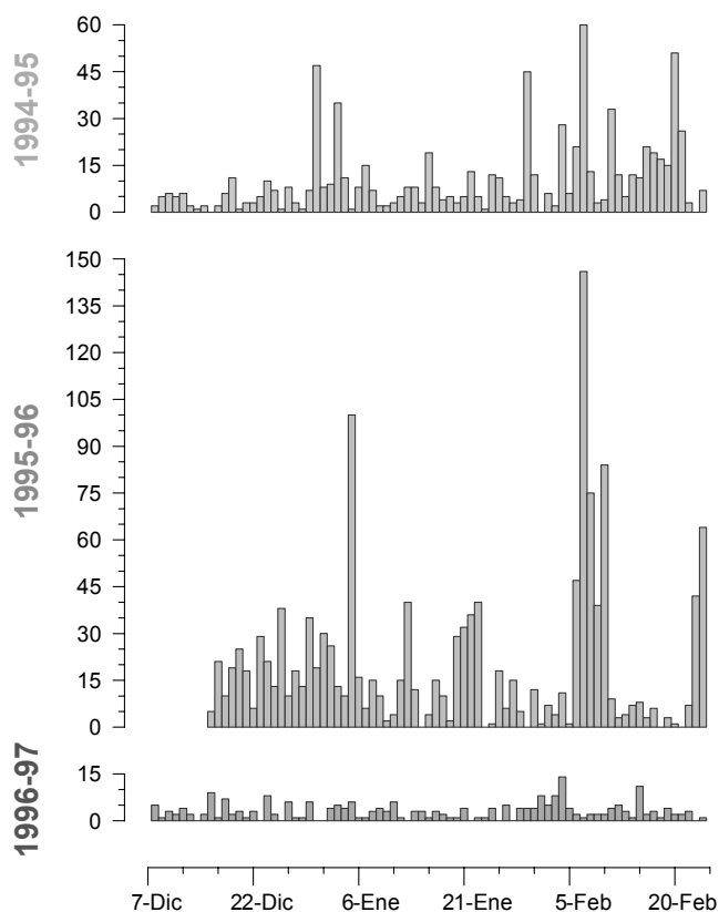
Figura 3.1. Número diario de eventos registrados por el array sísmico de la isla Decepción durante las tres campañas.
