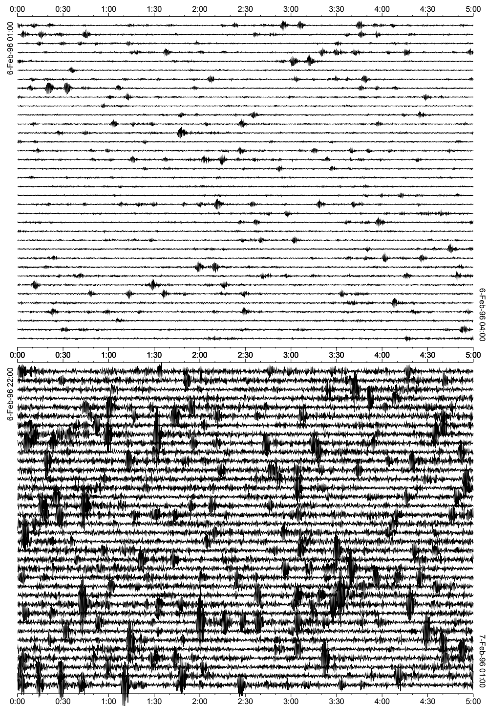
Figura 5.11. Ejemplos de registro continuo durante el enjambre de eventos de largo periodo ocurrido del 5 al 9 de febrero de 1996.
