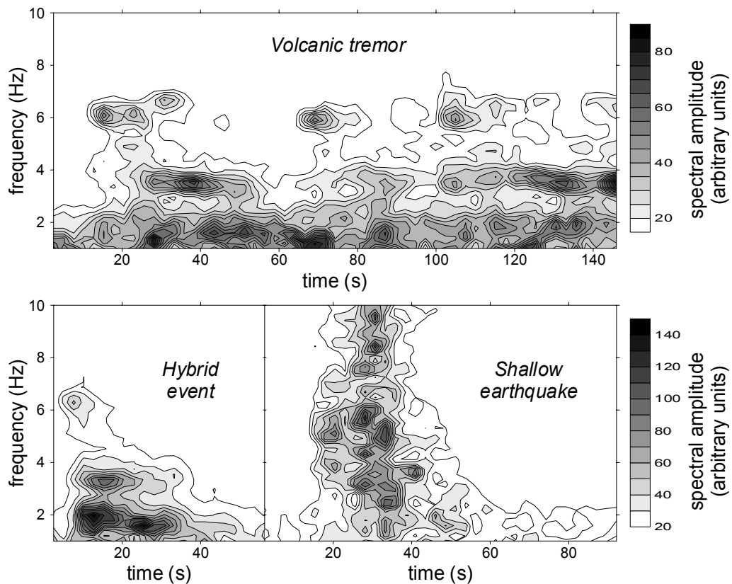
Figura 8.3. Comparación entre los espectrogramas de un tremor volcánico, un evento híbrido (registrados durante el periodo de actividad del 19 al 22 de enero de 1996) y un terremoto superficial (de ALMENDROS ET AL., 1997).
