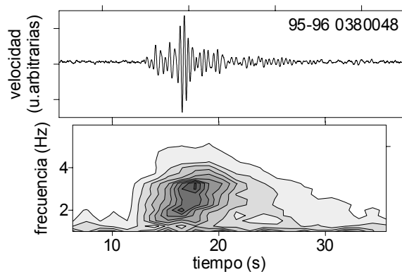
Figura 5.12. Sismograma de componente vertical y espectrograma promedio correspondiente para un evento de largo periodo LP2 típico, ocurrido durante la serie del 5 al 9 de febrero de 1996.
