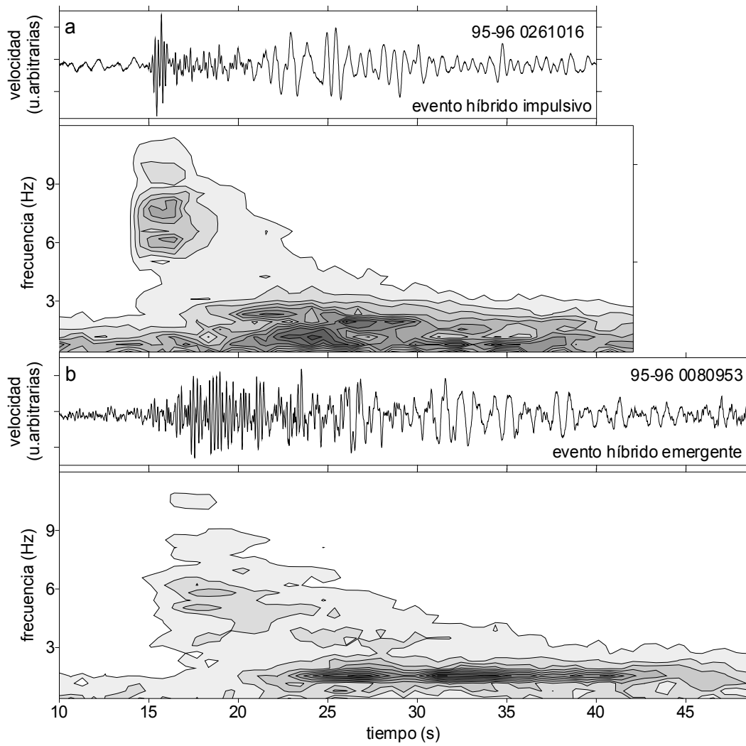
Figura 4.3. Sismogramas de componente vertical y espectrogramas promedio correspondientes para dos eventos híbridos de tipos HY (a) y HT (b). La llegada inicial de alta frecuencia queda perfectamente reflejada en los espectrogramas.
