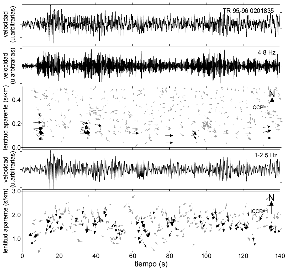
Figura 6.22. Resultados del método de la CCP a lo largo del tiempo para un tremor espasmódico TR. Obsérvese la llegada de paquetes de onda correlacionados en la banda de alta
