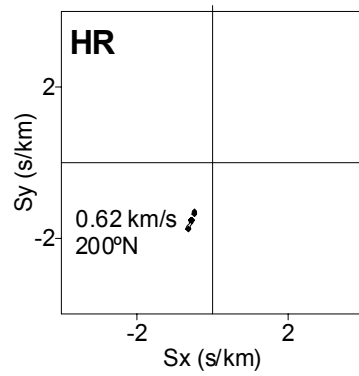
Figura 4.3. Resultados de la aplicación del método de alta resolución con una ventana de 2048 puntos.
