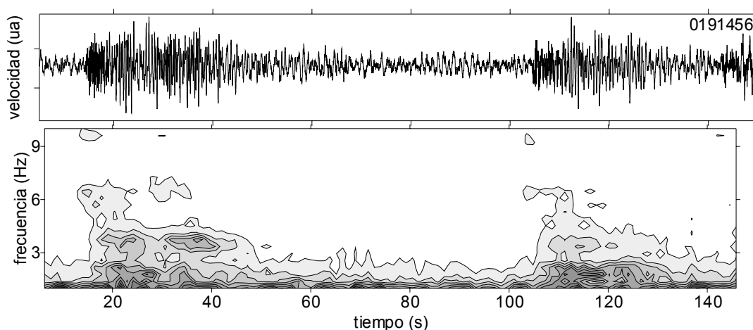
Figura 5.10. Sismograma de componente vertical y espectrograma promedio de una traza que contiene dos eventos híbridos HT que ocurren separados en el tiempo.
