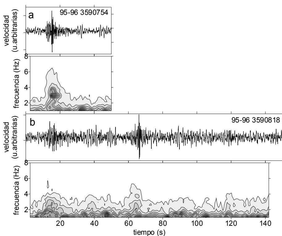
Figura 5.2. Sismogramas de componente vertical y espectrogramas promedio correspondientes para un evento de largo periodo (a) y un tremor (b), registrados durante el periodo de actividad del 25 de diciembre de 1995.
