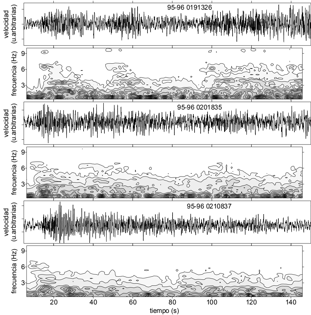
Figura 5.8. Trazas verticales y espectrogramas promedio de algunos de los tremores registrados durante el periodo de actividad de los días 19-22 de enero de 1996.
