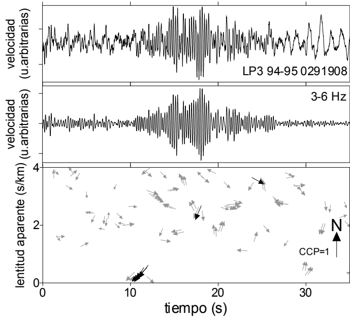
Figura 6.8. Representación de los resultados del análisis de la CCP a lo largo del tiempo para un evento de tipo LP3.
