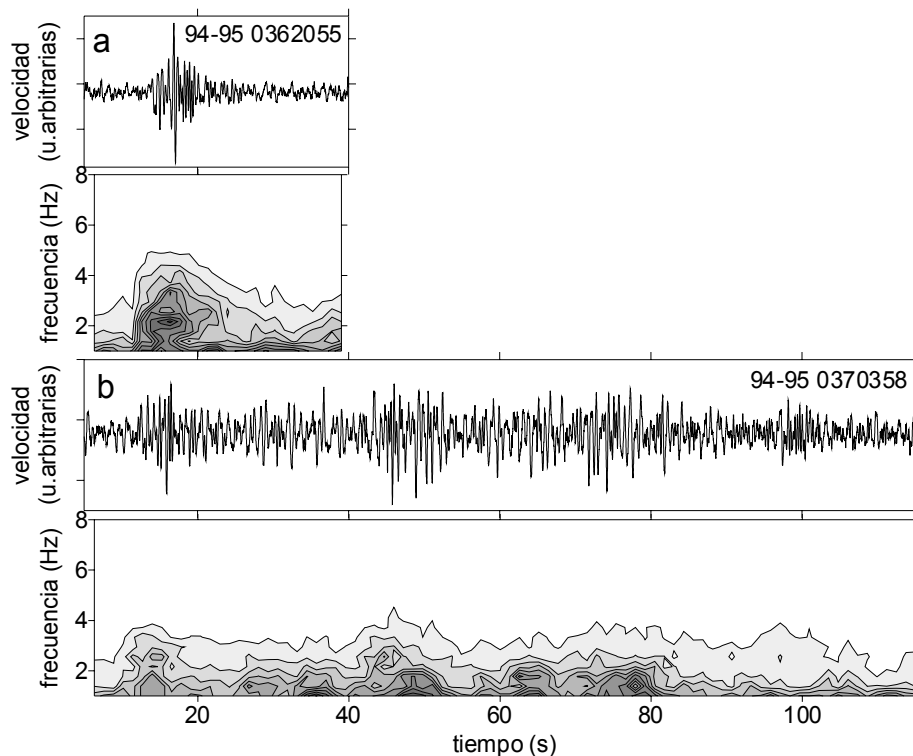
Figura 5.1. Sismogramas de componente vertical y espectrogramas promedio correspondientes para un evento de largo periodo (a) y un tremor volcánico (b) registrados durante el periodo de actividad del 5 al 7 de febrero de 1995.
