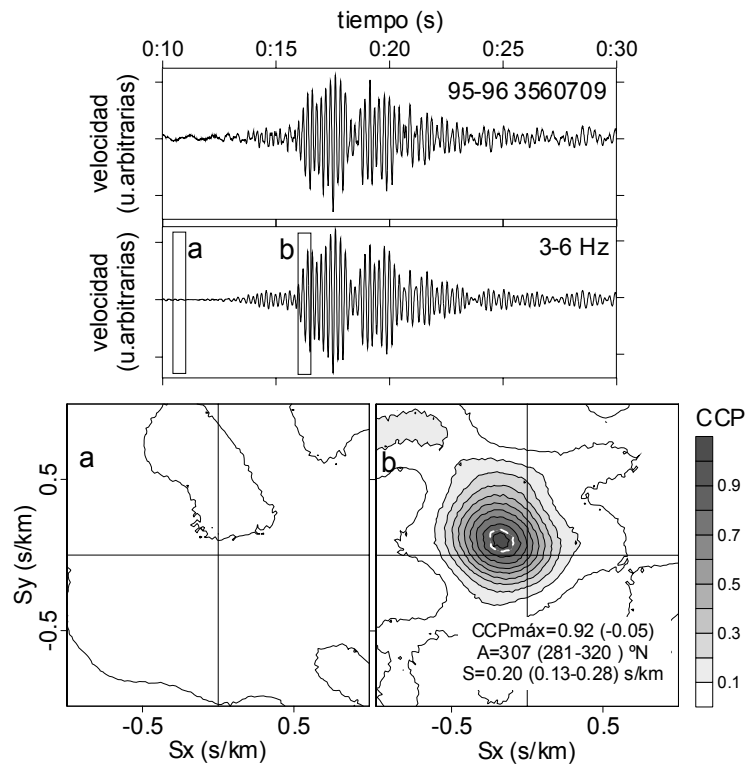
Figura 6.3. Igual que la Figura 6.2 para un evento de tipo LP3.
