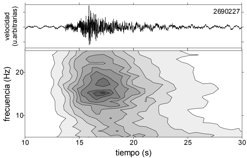
Figura 3.2. Sismograma de componente vertical (arriba) y espectrograma correspondiente (abajo) para un terremoto volcánico-tectónico.
