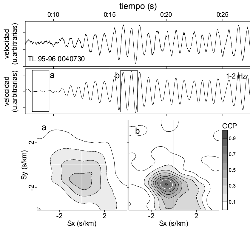
Figura 6.18. Igual que la Figura 6.2 para una porción de tremor volcánico de baja frecuencia.
