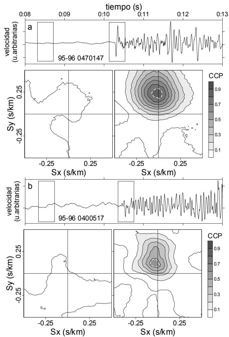
Figura 6.1. Resultado de la aplicación del método de la CCP para el ruido pre-evento y la primera llegada de la onda P de un terremoto local (a), y dos regionales (b y c). Posteriormente se verá que (b) es superficial y (c) es profundo.
