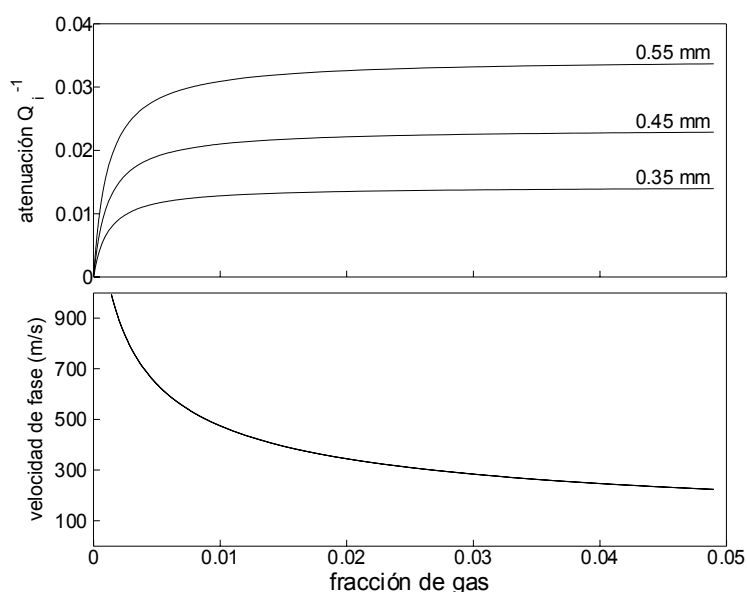
Figura 9.2. Atenuación y velocidad de fase en función del contenido en gas para distintos radios de las burbujas.
