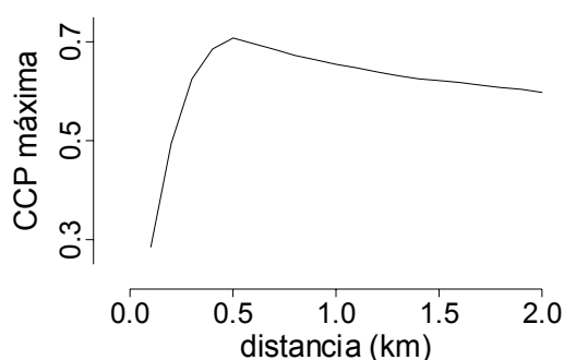
Figura 6.29. Representación de la CCP máxima en función de la distancia para el mismo evento analizado en la Figura 6.28.
