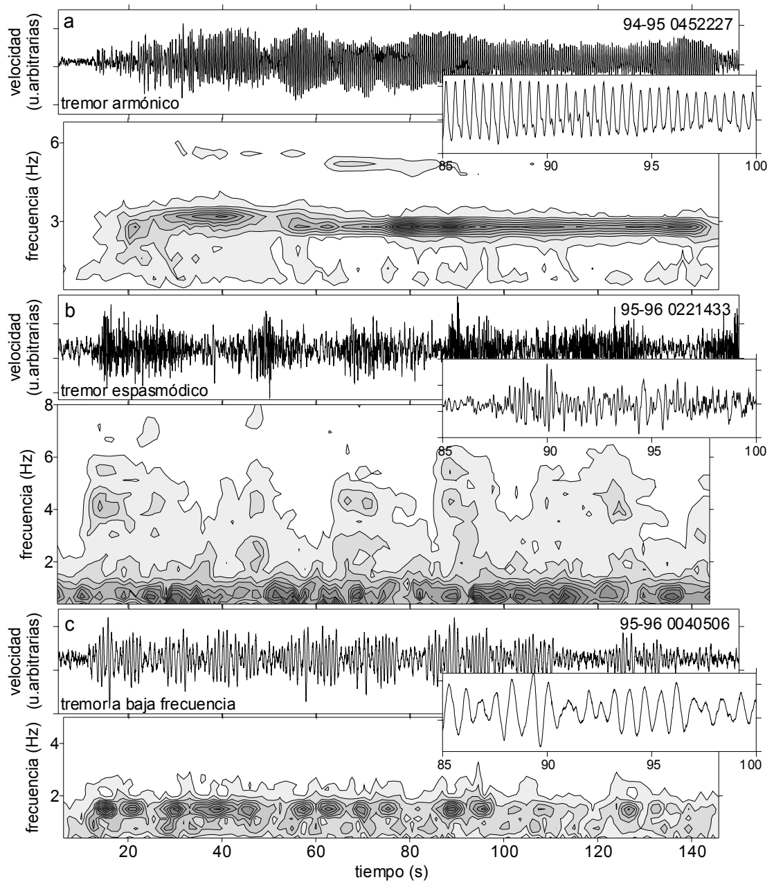
Figura 4.4. Sismogramas de componente vertical y espectrogramas promedio correspondientes para tremores volcánicos de los tipos armónico (a), espasmódico (b) y de baja frecuencia (c).
