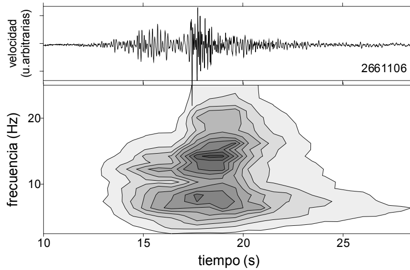
Figura 3.3. Sismograma de componente vertical (arriba) y espectrograma correspondiente (abajo) para una explosión, en la que se puede apreciar la llegada de la onda de aire.
