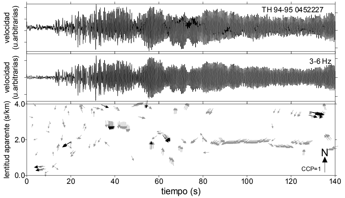
Figura 6.24. Resultados de la aplicación del método de la CCP a lo largo del tiempo para un tremor armónico TH.
