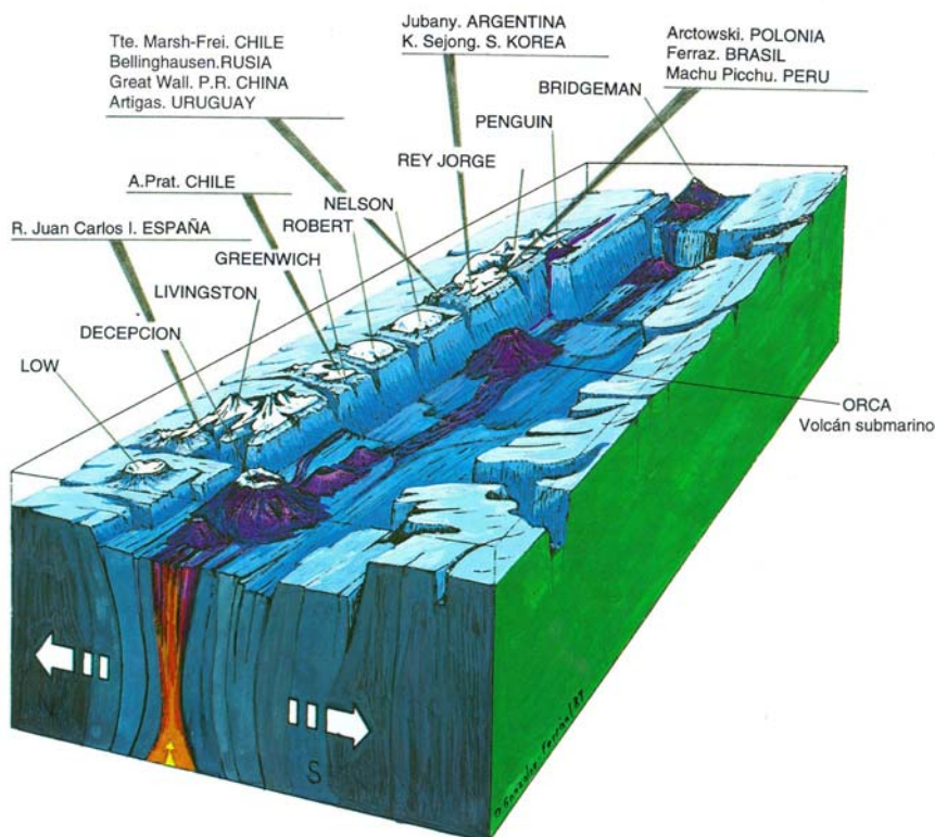
Figura 1.2. Esquema del rift de Bransfield, en el que aparece la cadena volcánica a la que pertenece Decepción (de GONZÁLEZ FERRÁN, 1995).
