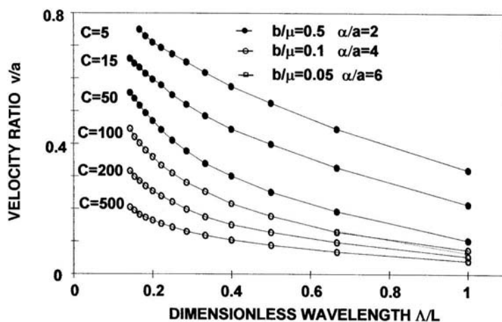
Figura 9.3. Razón entre la velocidad del medio y la del fluido (de GIL CRUZ & CHOUET, 1997)
