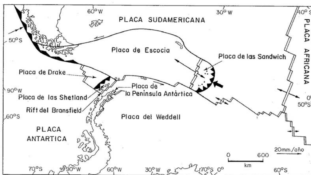
Figura 1.1. Esquema tectónico alrededor del estrecho de Bransfield y las islas Shetland del Sur (de GONZÁLEZ FERRÁN, 1995).
