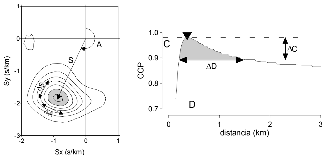
Figura 4.7. Esquema del procedimiento para la determinación del error en el método de la CCP.
