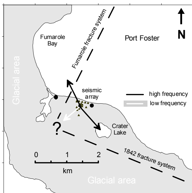
Figura 6.26. Esquema de las posibles zonas responsables de la actividad sismo-volcánica registrada por el array de la isla Decepción.
