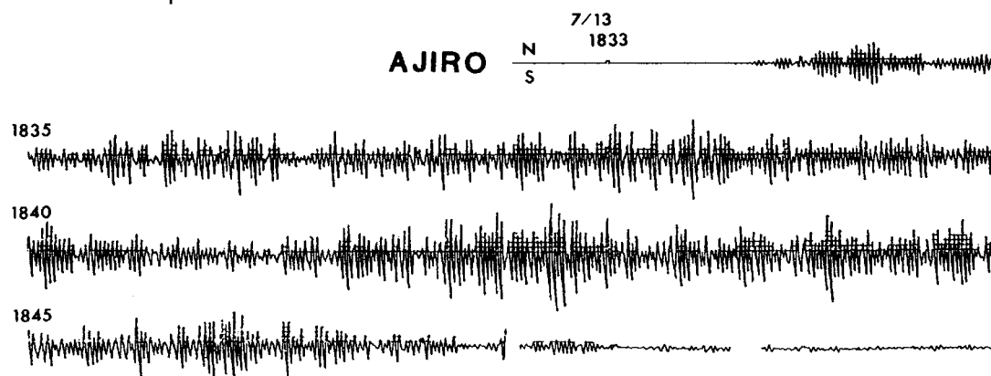
Figura 2.5. Episodio de tremor volcánico registrado el 13 de julio de 1989, durante la erupción submarina junto a la península de Izu (Japón). El registro corresponde a la componente NS de un sensor de 5 s de periodo natural (GOTO ET AL., 1991).
