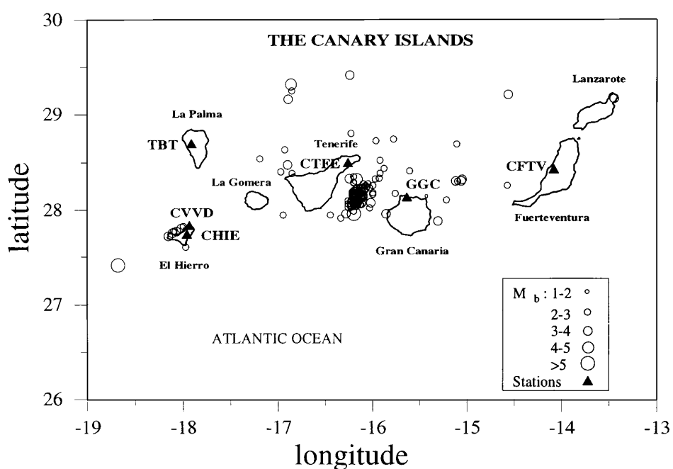
Figura 1.4. Distribución de epicentros de los terremotos registrados por la red sísmica del Instituto Geográfico Nacional (de CANAS ET AL., 1998)
