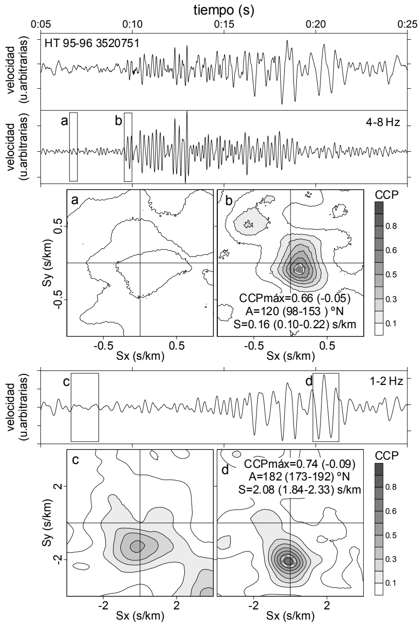
Figura 6.12. Igual que la Figura 6.2 para un evento híbrido HT.
