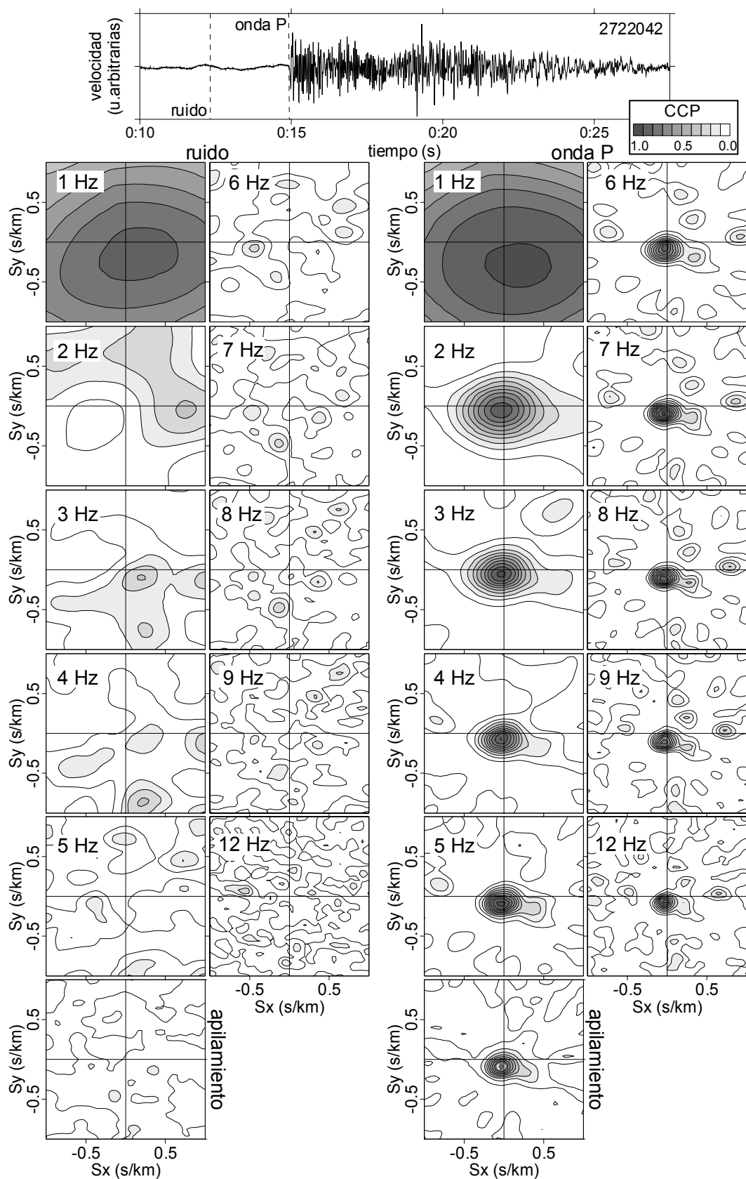
Figura 4.1. Resultados del análisis de la CCP sobre el plano de lentitud aparente para el ruido pre-evento y la llegada de la onda P de un terremoto tectónico local.
