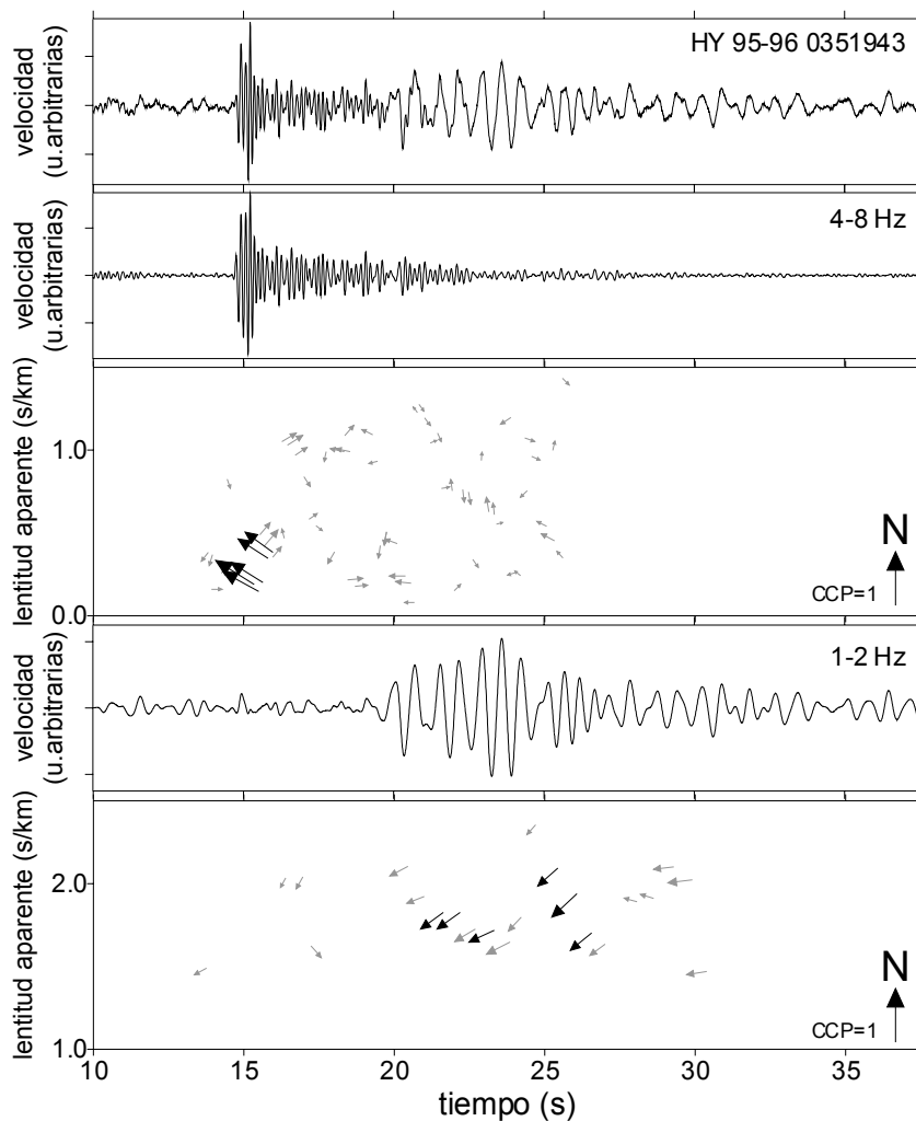
Figura 6.13. Variación de los resultados del análisis de la CCP a lo largo del tiempo par un evento híbrido HY.
