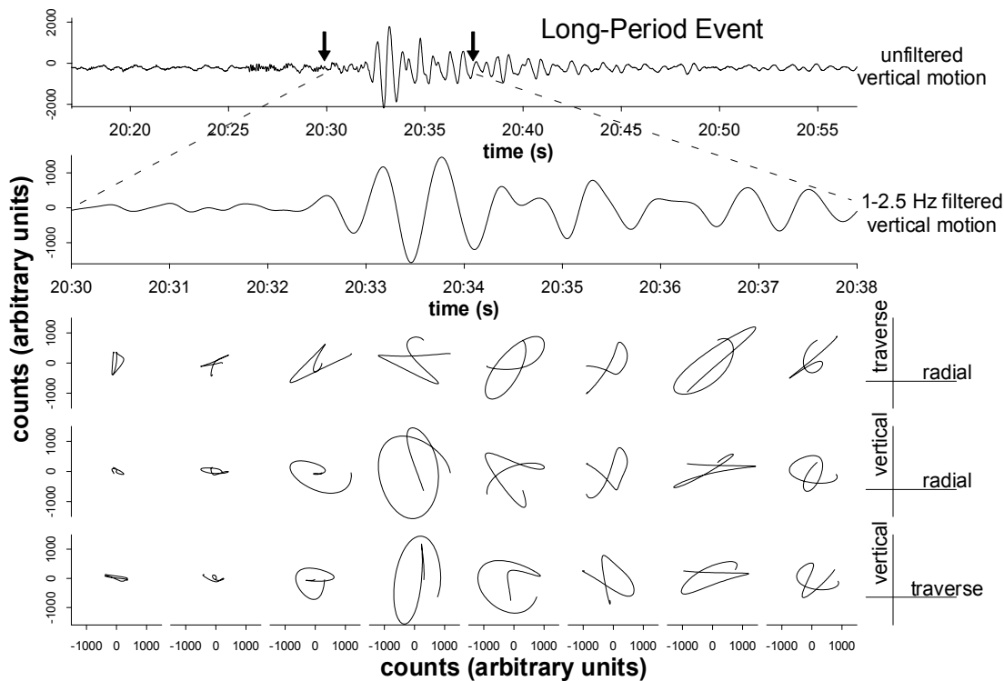
Figura 7.1. Movimiento de la partícula para las ondas de baja frecuencia que componen los eventos de largo periodo (de DEL PEZZO ET AL., 1998).
