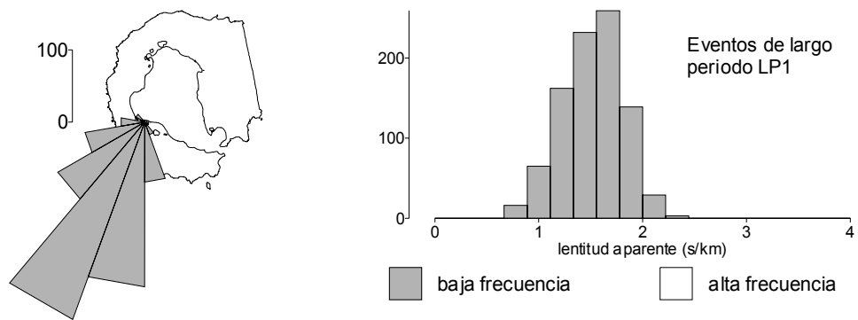
Figura 6.5. Histograma de los resultados obtenidos para todos los eventos de largo periodo de tipo LP1.
