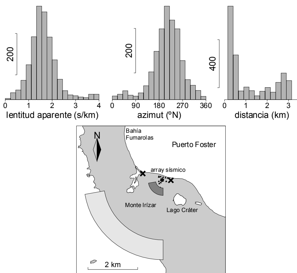
Figura 6.32. (arriba) Histogramas de lentitud aparente, azimut y distancia para todas las soluciones obtenidas a lo largo de los distintos eventos analizados. (abajo) Mapa en el que se muestra la zona fuente más probable (el sector oscuro) y la correspondiente al máximo secundario a 2.8 km (el sector claro).
