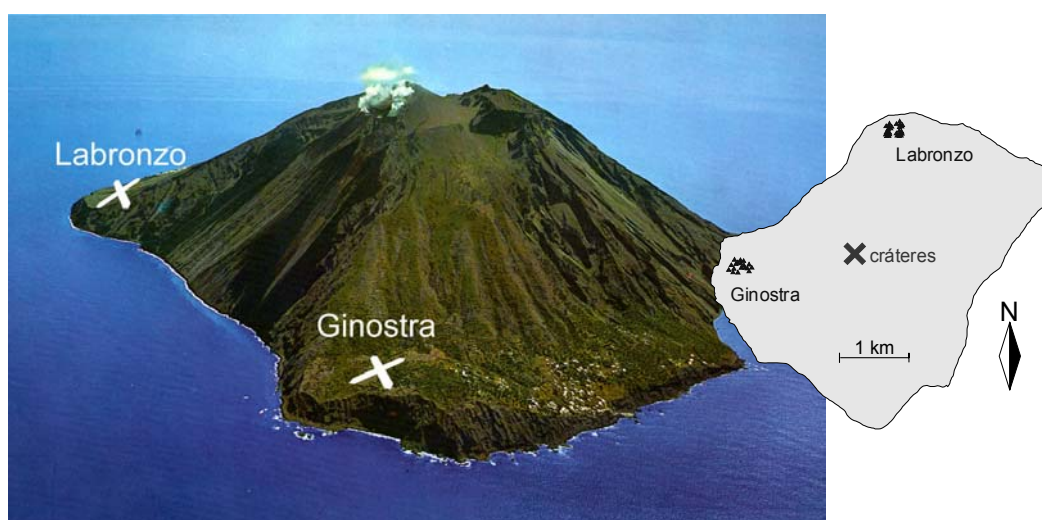
Figura 2.1. Situación de los arrays sísmicos en la isla.
