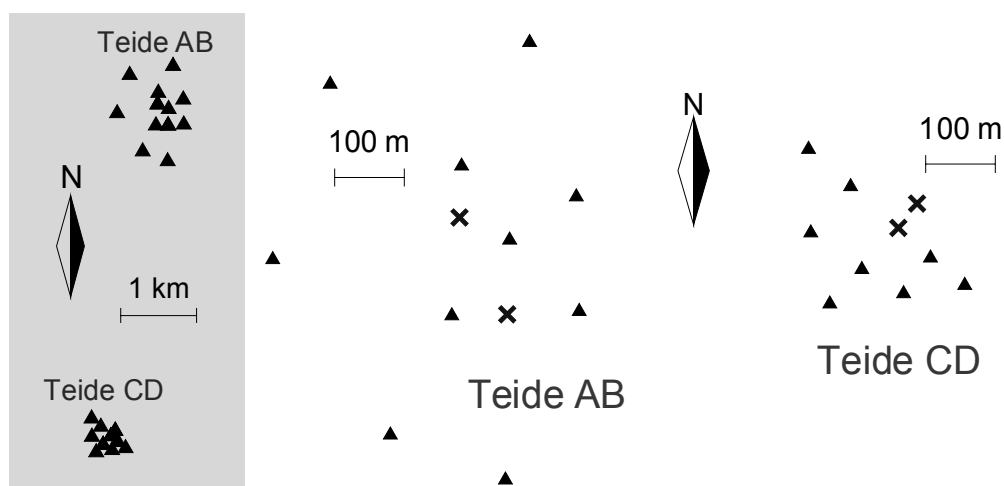
Figura 2.2. Situación relativa de los arrays sísmicos utilizados en el experimento (izquierda) y configuración correspondiente (derecha). Los triángulos representan las estaciones verticales, y las espas las de tres componentes.
