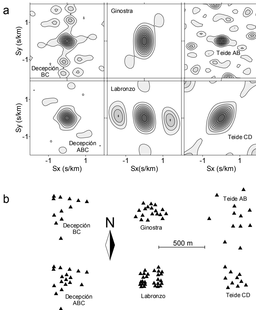
Figura 4.4. Patrón de antena para el método BF (a) de todas las configuraciones del array utilizadas en la presente tesis (b).
