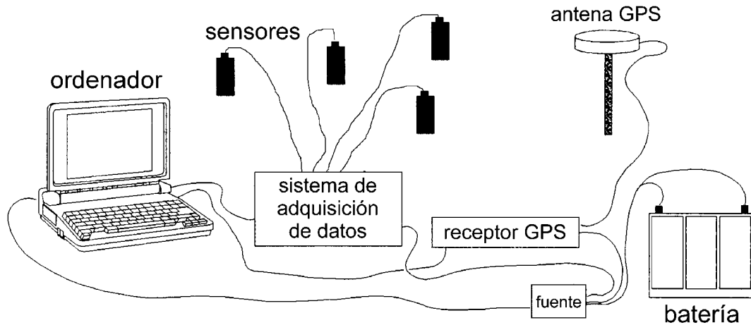
Figura 2.1. Esquema de los componentes fundamentales del array sísmico (modificado de ORTIZ ET AL., 1994A).
