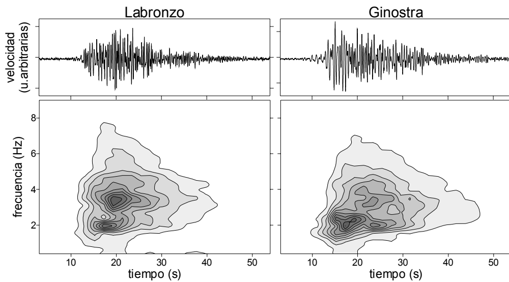
Figura 3.1. Sismogramas de componente vertical y espectrogramas de una explosión característica registrada en los arrays de Labronzo y Ginostra.
