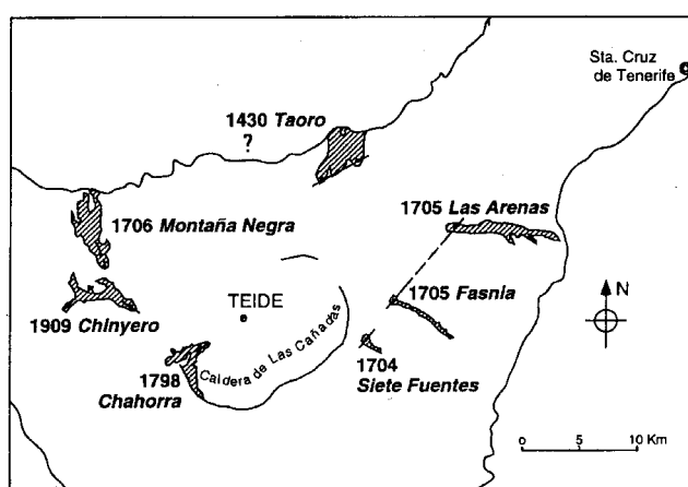
Figura 1.3. Localización de las erupciones históricas más recientes ocurridas en la isla de Tenerife (de MARTÍ ET AL., 1994).
