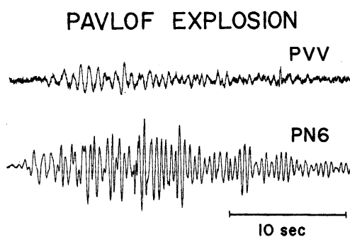
Figura 2.4. Ejemplo de una explosión volcánica en el volcán Pavlof (de McNUTT, 1986).
