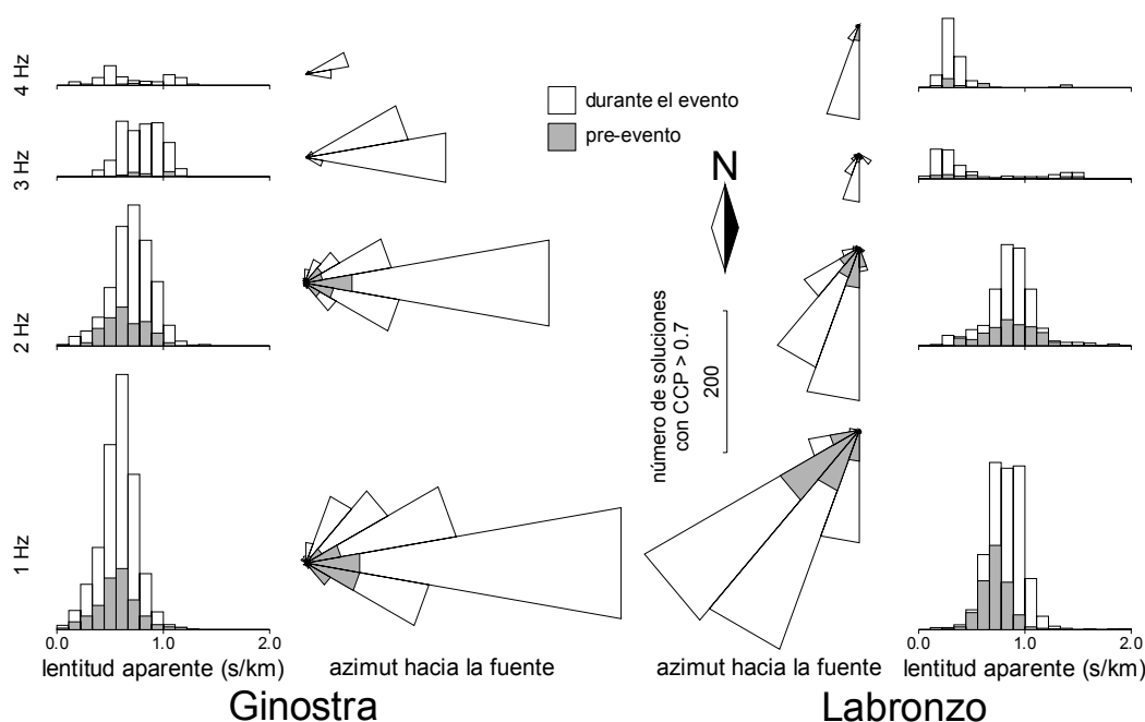
Figura 4.4. Comparación entre las soluciones con buena correlación (CCP mayor de 0.7) obtenidas para el ruido pre-evento (gris) y durante las explosiones (blanco).
