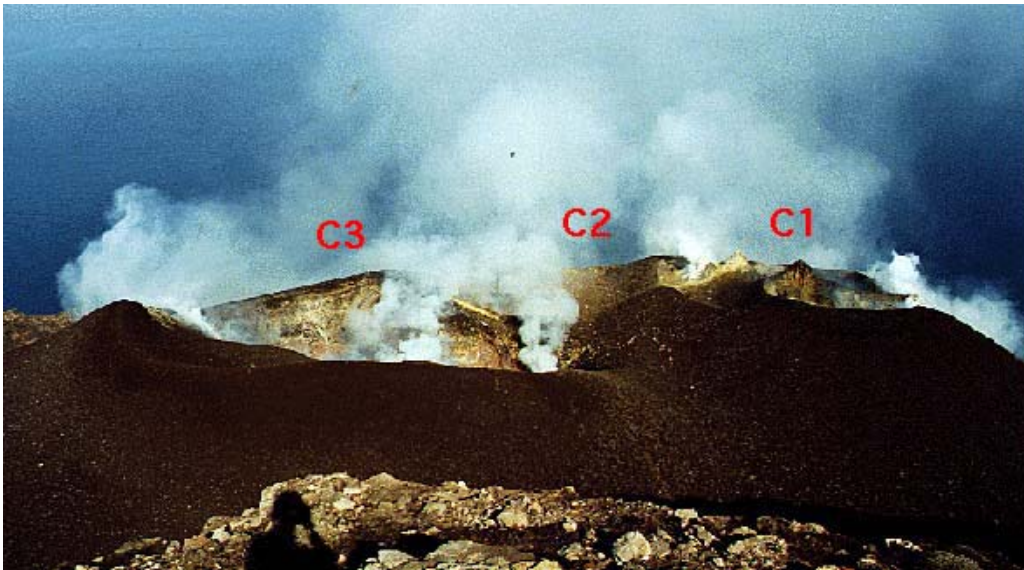
Figura 1.3. Vista hacia el noroeste desde la cumbre de Stromboli. Puede apreciarse la presencia de tres cráteres activos, marcados como C1, C2 y C3.
