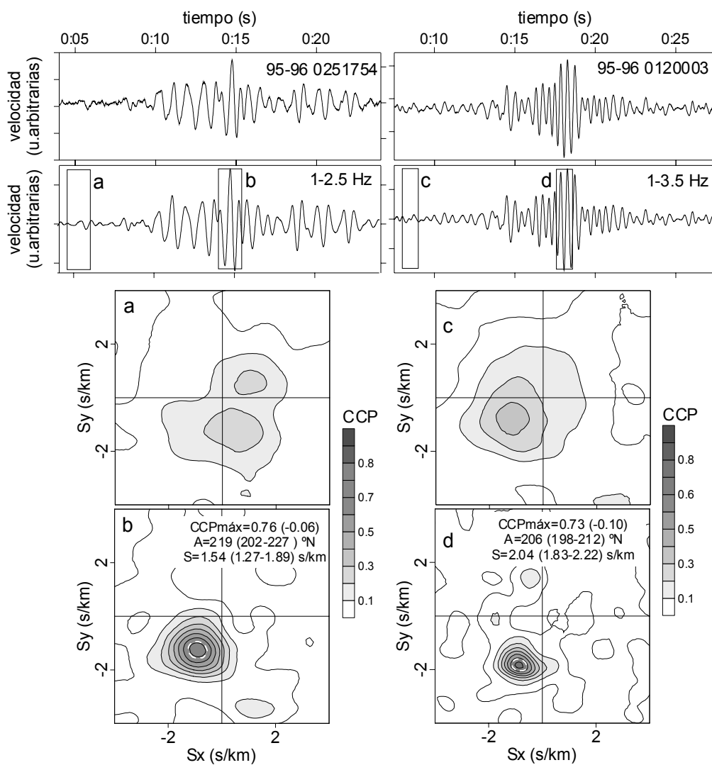
Figura 6.2. Resultado de la aplicación del método de la CCP a eventos de largo periodo de tipos LP1 (izquierda) y LP2 (derecha). En ambos casos, la primera ventana corresponde al ruido pre-evento (a y c), mientras que la segunda es la que da la mayor CCP de toda la señal (b y d), y se toma como localización del evento. Los resultados incluyen la CCP máxima, el azimuth hacia la fuente y la lentitud aparente, junto a sus intervalos de error.
