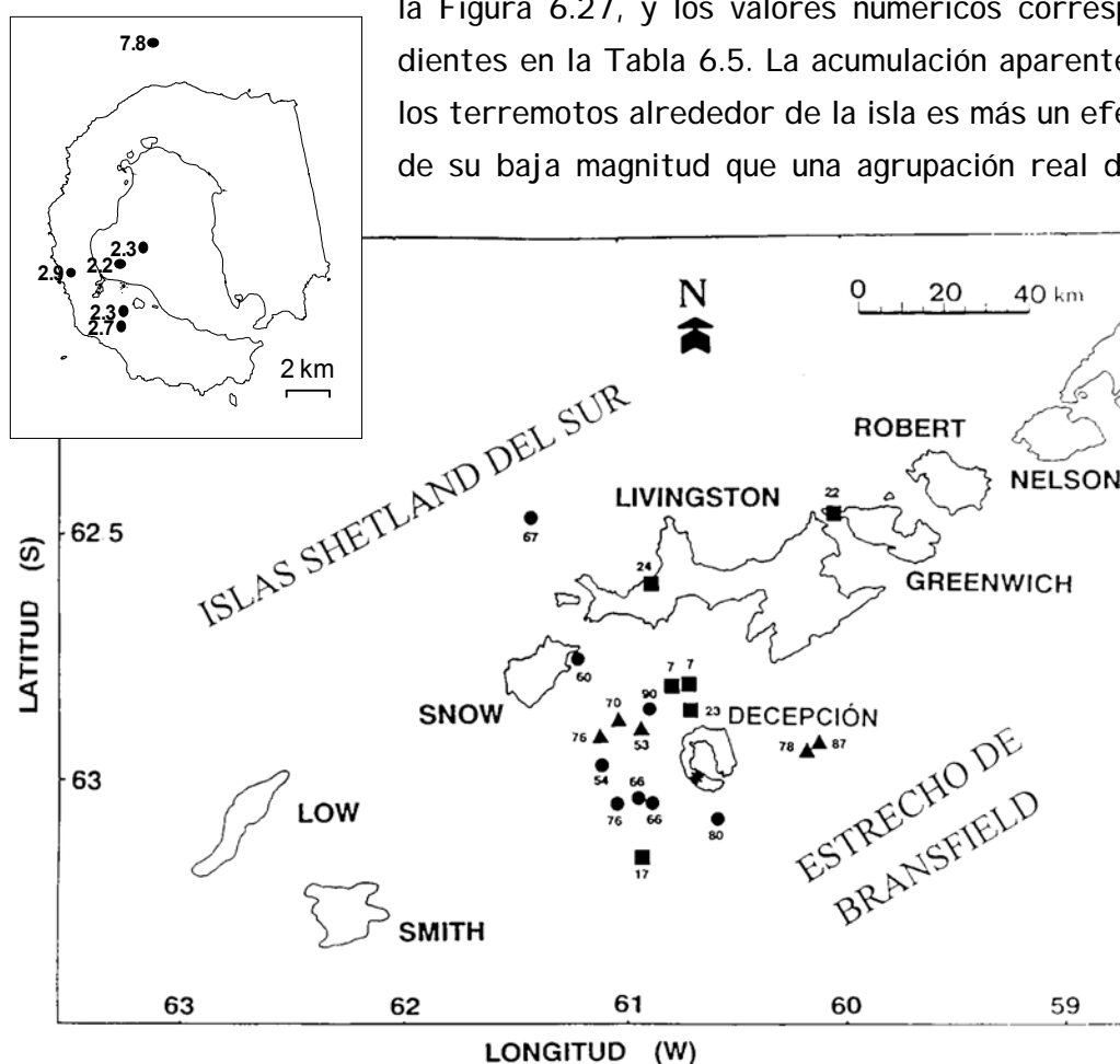
Figura 6.27. Situación de los epicentros de los terremotos localizados mediante el trazado inverso del rayo. El número junto a los símbolos representa la profundidad en km (modificado de IBAÑEZ ET AL., 1997).
