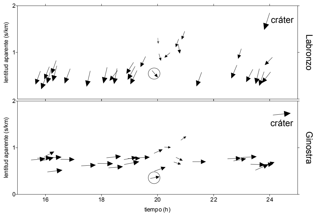
Figura 4.3. Representación de los resultados de la localización utilizando los arrays de Labronzo y Ginostra. Los valores numéricos se muestran en la Tabla 4.2. El círculo indica la ocurrencia del terremoto volcano-tectónico que se discute en el texto.
