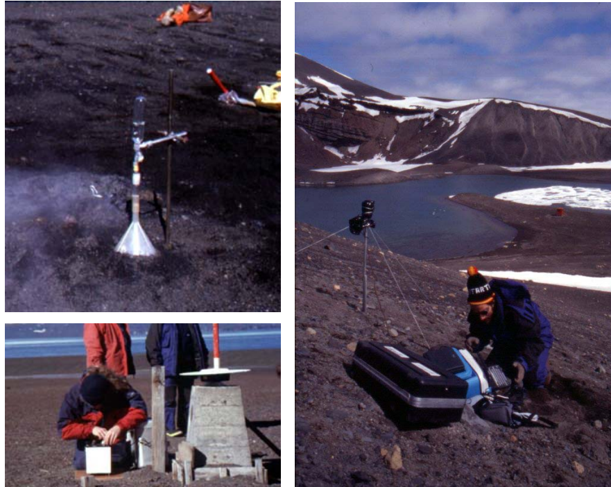
Figura 4.27. Algunos de los proyectos geofísicos que se desarrollaron en la isla Decepción durante las campañas antárticas: medidas del campo magnético (derecha), gravimetría y geodesia (izquierda abajo) y estudios de geoquímica de gases (izquierda arriba).
