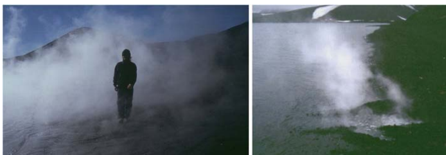
Figura 1.5. (izquierda) Nubes de vapor de agua producidas por la evaporación sobre una zona caliente en Caleta Péndulo. (derecha) Emisión de gases de una fumarola en Bahía Fumarolas.
