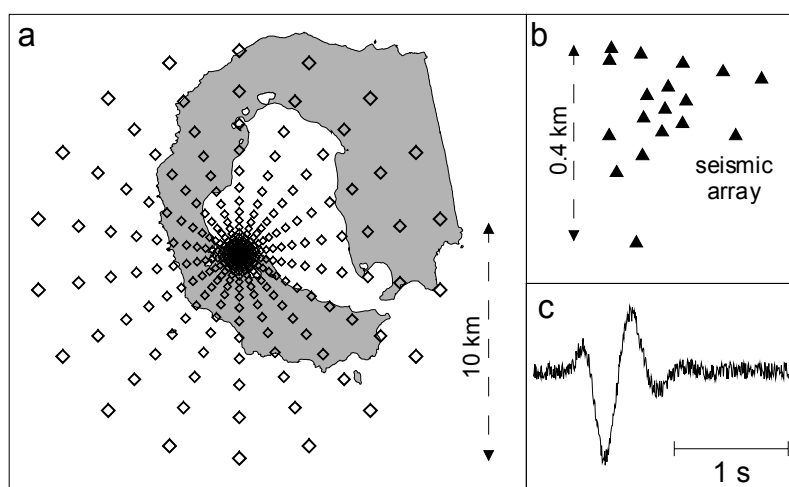
Figura 4.6. (a) Mapa de la isla Decepción, sobre el que se han situado los epicentros considerados en el test. (b) Configuración del array sísmico de la isla Decepción, con el que se han localizado las señales. (c) Forma del pulso empleado.
