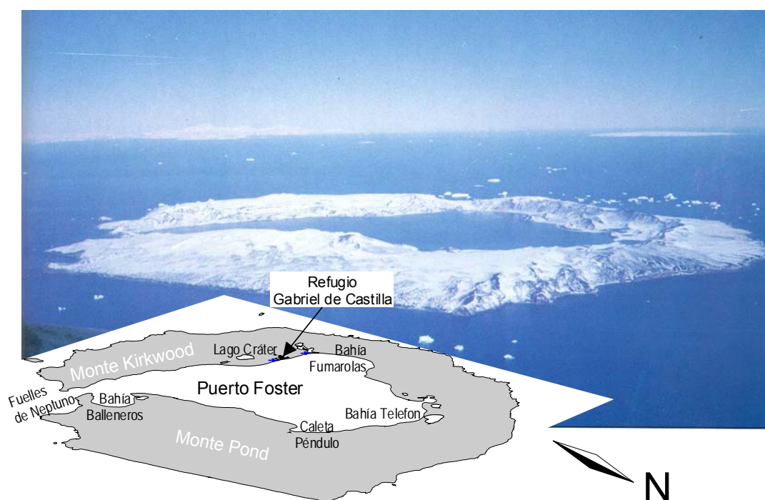
Figura 1.4. Vista aérea de la isla Decepción. En el esquema se señalan algunos topónimos citados en el texto. La flecha indica la posición de la Base Gabriel de Castilla.
