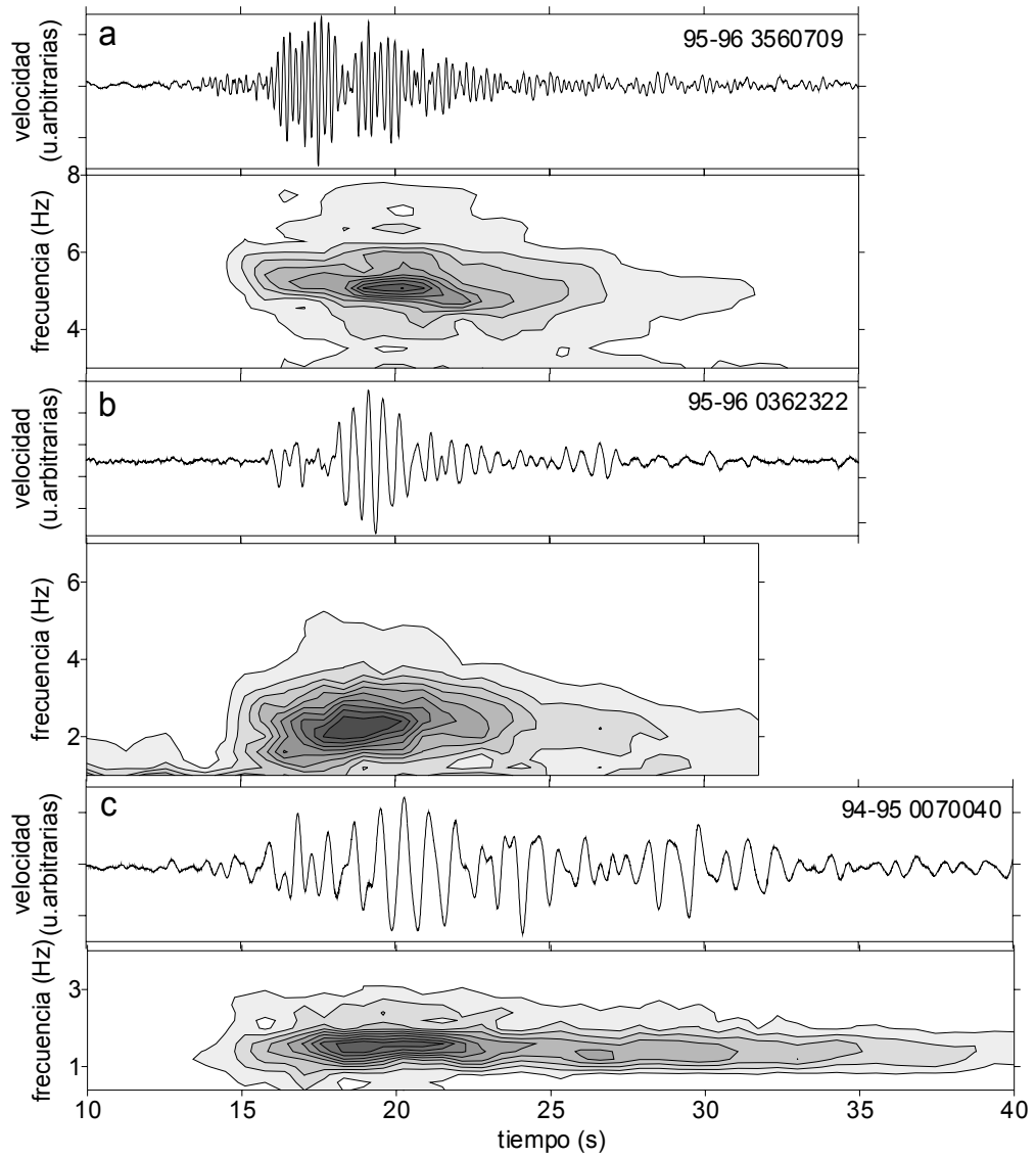
Figura 4.2. Sismogramas de componente vertical de tres eventos de larga frecuencia de los tipos LP3 (a), LP2 (b) y LP1 (c), y espectrogramas promedio correspondientes. Obsérvese que el contenido espectral se reduce a una estrecha banda de frecuencia.
