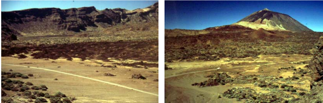
Figura 4.2. Vista del Teide y de la caldera de Las Cañadas desde la zona del array .
