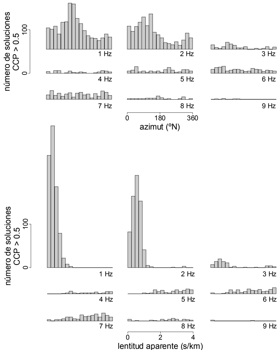
Figura 4.4. Histograma de las soluciones con CCP mayor de 0.5 encontradas en el análisis del ruido, para las distintas bandas de frecuencia, en función del azimut (arriba) y la lentitud aparente (abajo).
