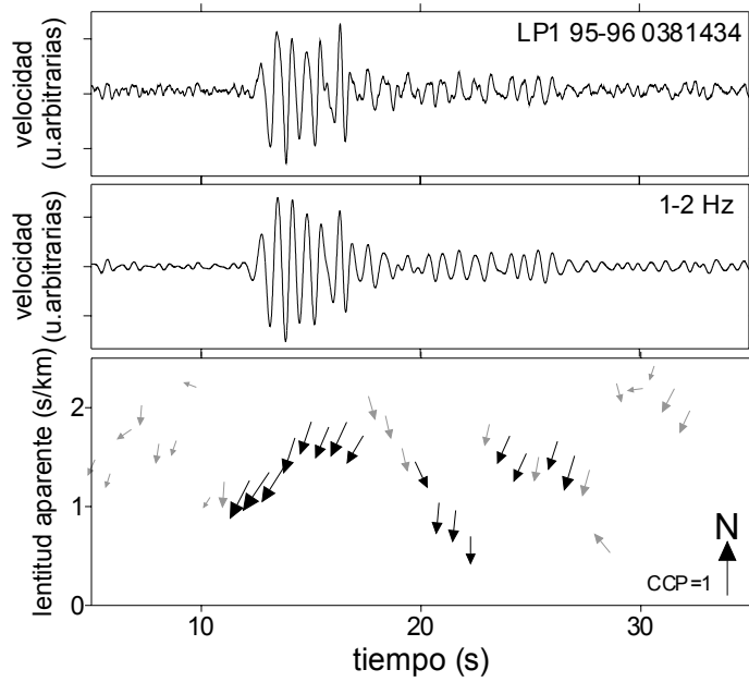
Figura 6.4. Representación de los resultados del análisis de la CCP a lo largo del tiempo para un evento de largo periodo de tipo LP1.
