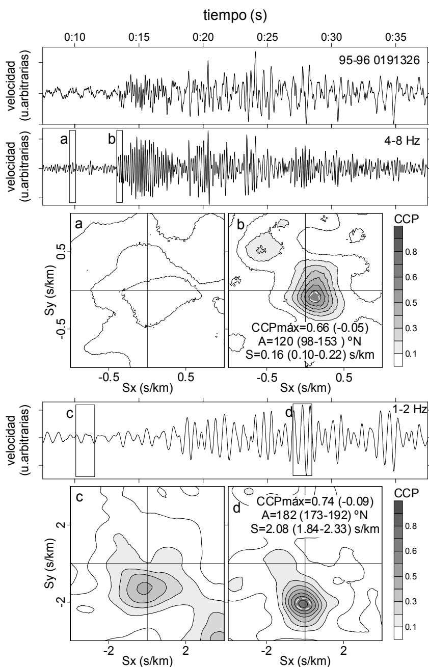
Figura 6.17. Igual que la Figura 6.2 para un tremor volcánico TR. El análisis se realiza por separado por las dos bandas de frecuencia.
