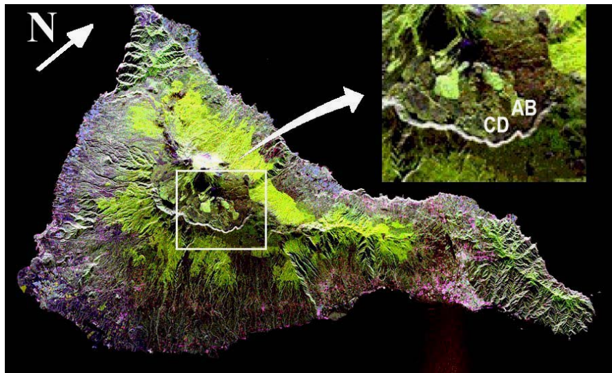
Figura 2.1. Imagen de satélite de la isla de Tenerife. Puede apreciarse el cráter del Teide, casi en el centro de la isla, y el borde de la caldera de las Cañadas. La posición de los arrays se indica en la zona ampliada.
