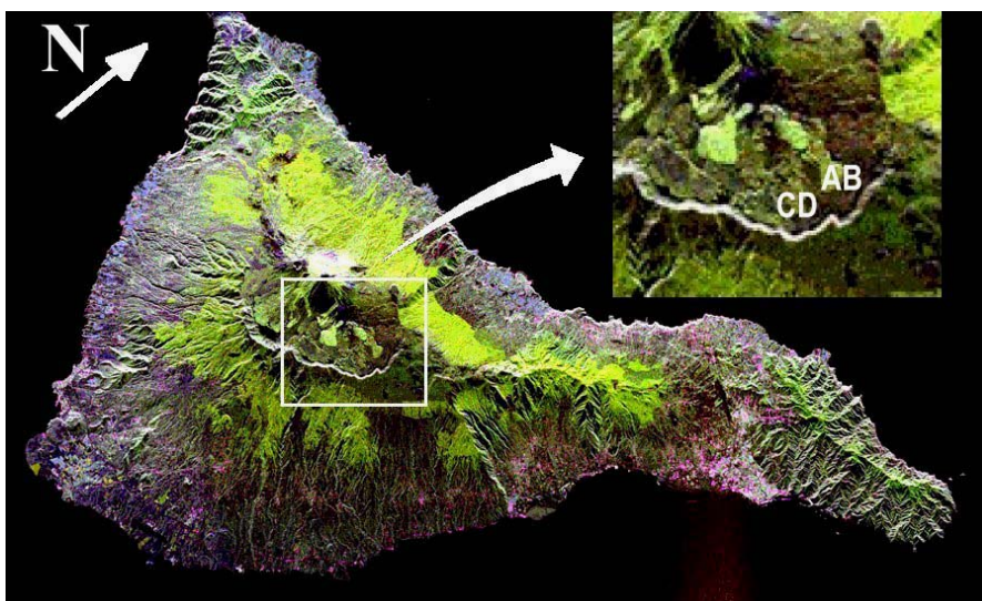
Figura 4.1. Imagen de satélite de la isla de Tenerife. Puede apreciarse el cráter del Teide, casi en el centro de la isla, y el borde de la caldera de las Cañadas. La posición de los arrays se indica en la zona ampliada.
