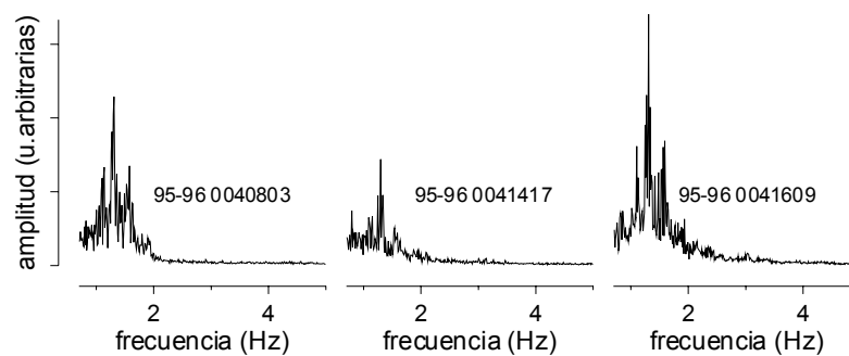
Figura 5.6. Amplitud espectral de las porciones de tremor de la Figura 5.5. Obsérvese la constancia del pico espectral a 1.3 Hz durante toda la serie.
