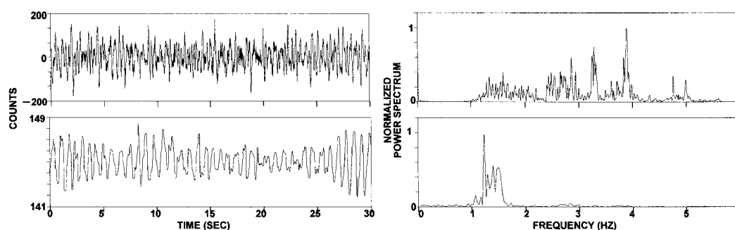
Figura 2.6. Ejemplos de tremor volcánico registrado en el volcán Galeras (Colombia) durante la actividad eruptiva de mayo de 1989. Se muestra una porción de las trazas de la componente vertical (izquierda) junto con el espectro correspondiente (derecha). Puede verse que el segundo tiene un contenido espectral mucho más restringido (GIL CRUZ & CHOUET, 1997).
