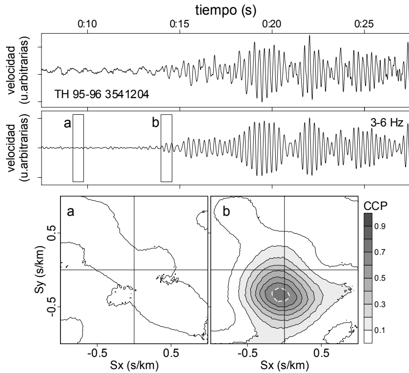
Figura 6.19. Igual que la Figura 6.2 para el comienzo de un tremor armónico TH.
