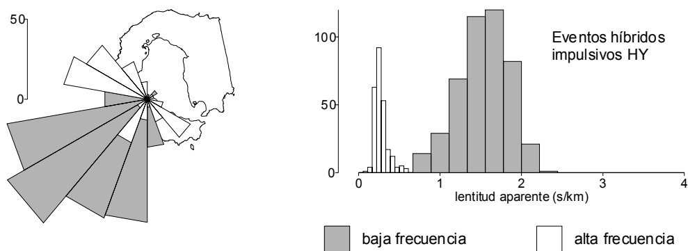
Figura 6.14. Histograma de los resultados obtenidos para todos los eventos híbridos de tipo HY.
