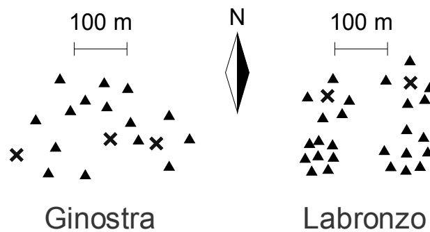
Figura 2.2. Configuración de los arrays sísmicos empleados.
