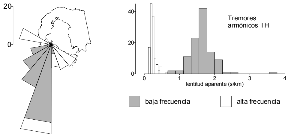
Figura 6.25. Histogramas de los resultados obtenidos para todos los tremores armónicos.
