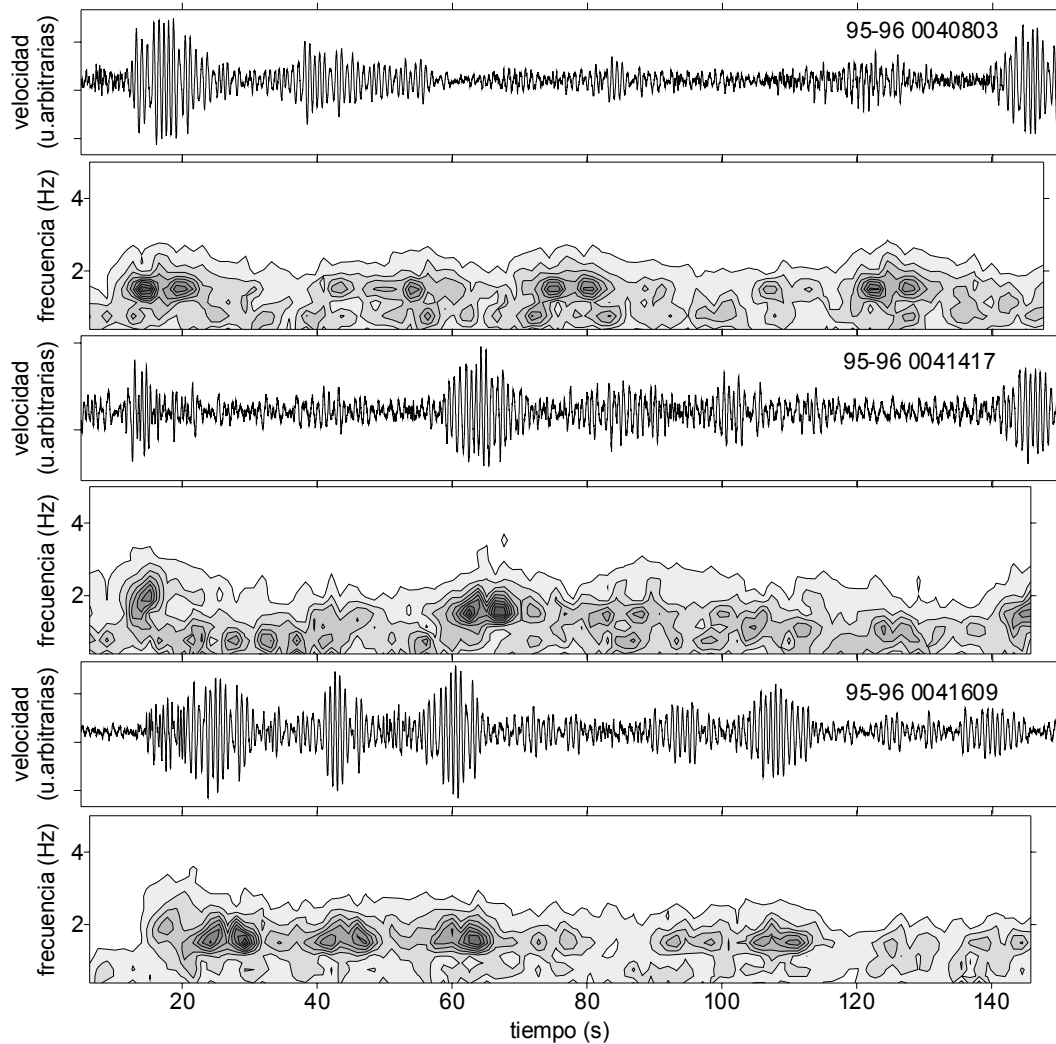
Figura 5.5. Porciones de tremor registradas durante el periodo de actividad ocurrido el 4 de enero de 1996, junto con los correspondientes espectrogramas promedio.
