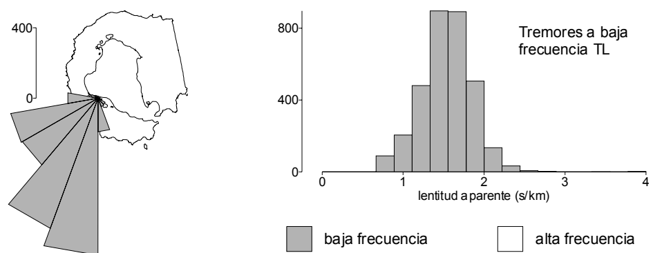
Figura 6.20. Resultados del método de la CCP a lo largo del tiempo para un episodio de trémor de baja frecuencia TL.
