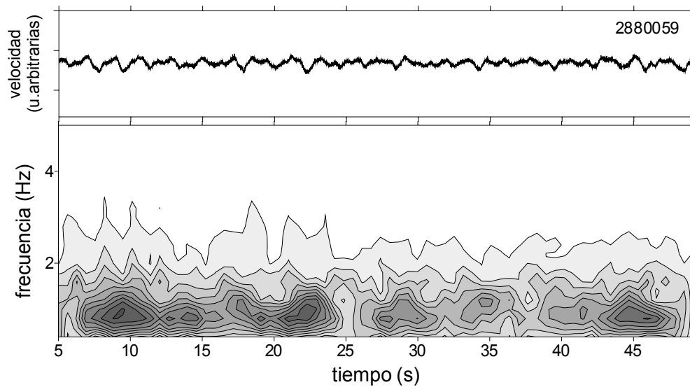
Figura 3.4. Muestra de la componente vertical de uno de los registros de ruido (arriba) y espectrograma correspondiente (abajo).
