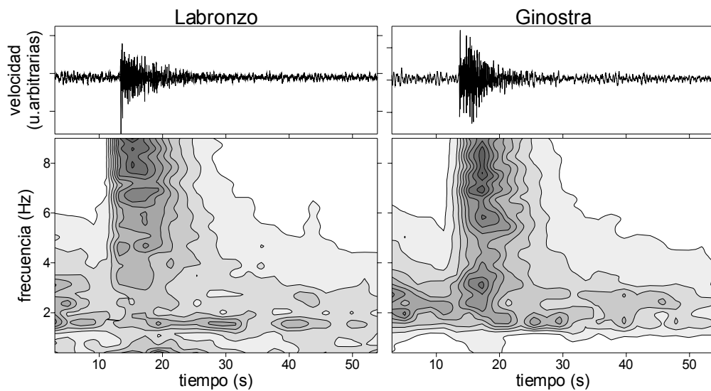
Figura 3.2. Sismogramas de componente vertical y espectrograma de un terremoto tectónico local registrado en los arrays de Labronzo y Ginostra.
