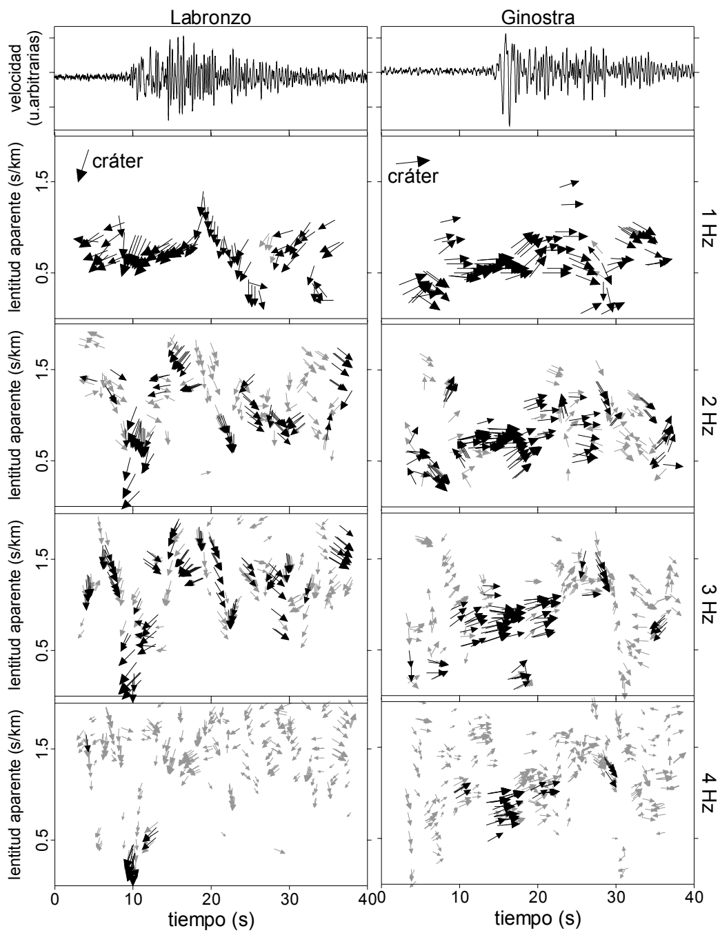
Figura 4.2. Variación temporal de la localización de una de las explosiones estudiadas.
