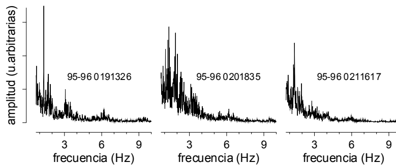
Figura 5.9. Amplitud espectral correspondiente a las porciones de tremor que aparecen en la Figura 5.8.
