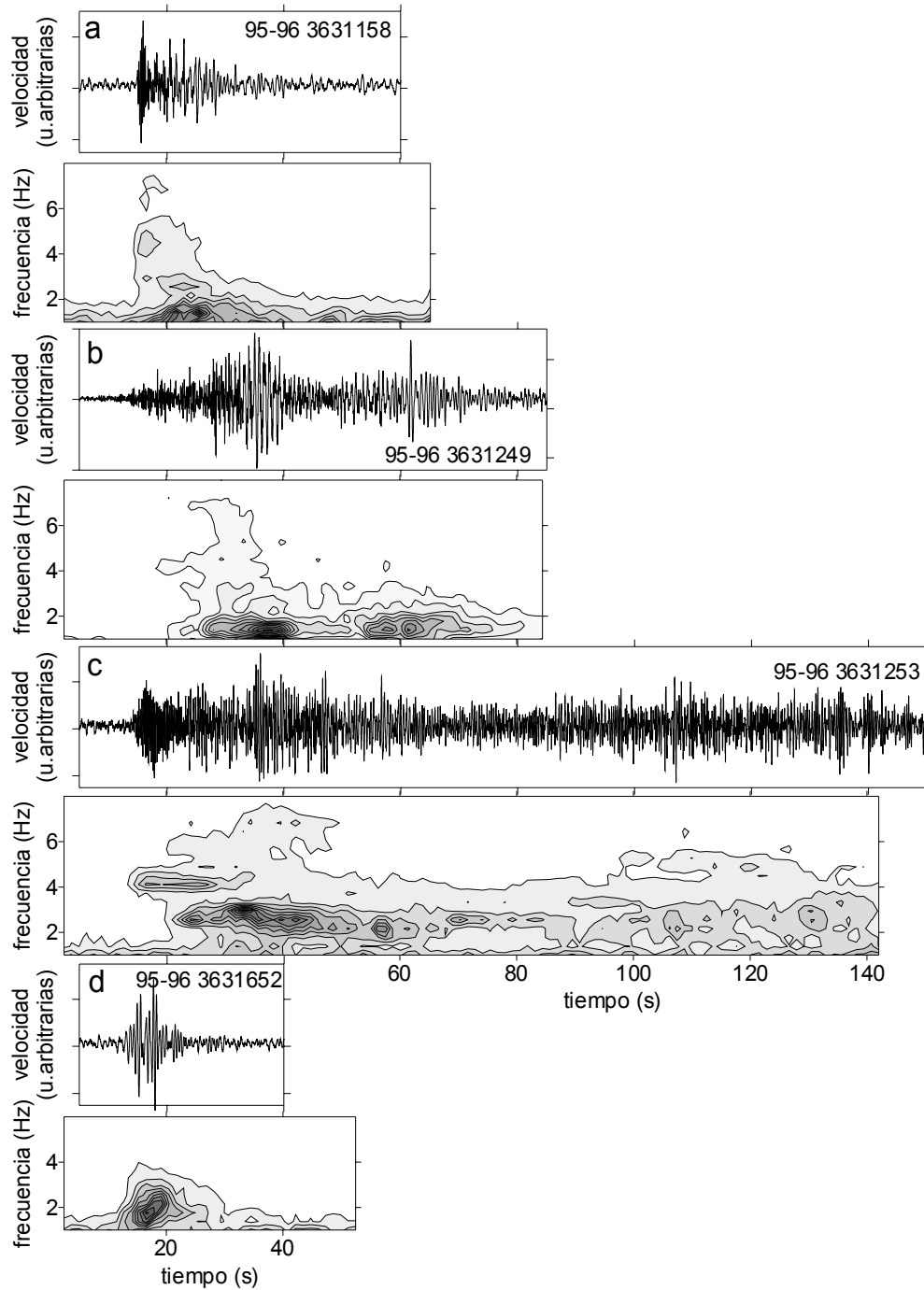
Figura 5.3. Sismogramas de componente vertical y espectrogramas correspondientes para un evento híbrido HY (a), otro HT (b), un tremor (c) y un evento de largo periodo (d), registrados durante el periodo de actividad del 29 de diciembre de 1995.
