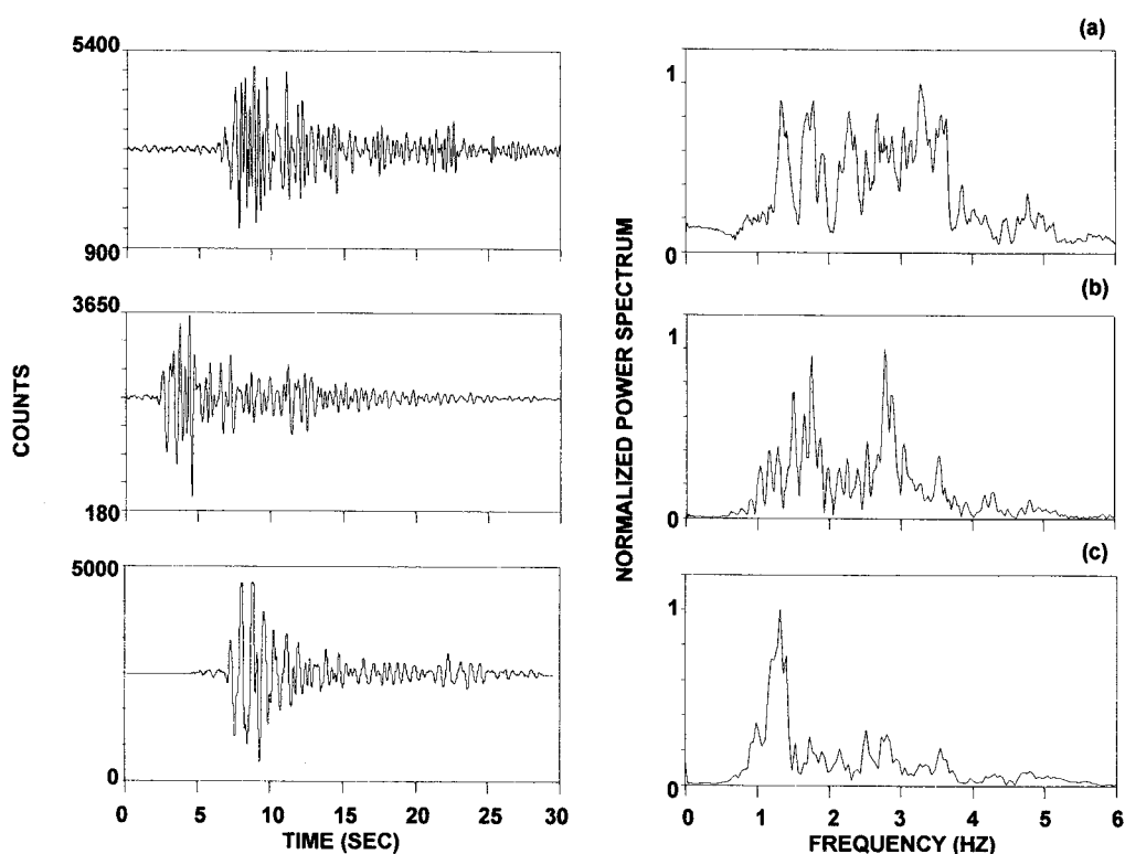
Figura 2.2. (Izquierda) Eventos de largo periodo registrados en el volcán Galeras durante la extrusión de un domo de lava en 1991. (Derecha) Espectro correspondiente. (GIL CRUZ & CHOUET, 1997).
