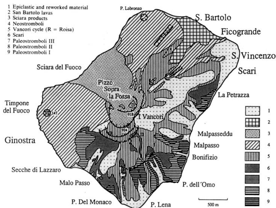
Figura 1.2. Esquema geológico de Stromboli, mostrando la distribución de las principales unidades estratigráficas (de HORNIG-KJARSGAARD ET AL., 1993).
