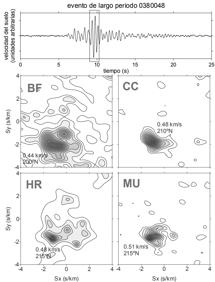
Figura 4.5. Resultados de la aplicación de los cuatro métodos citados en el texto a la localización de un evento de largo periodo. En km/s se da la velocidad aparente, y en °N el azimut hacia la fuente.
