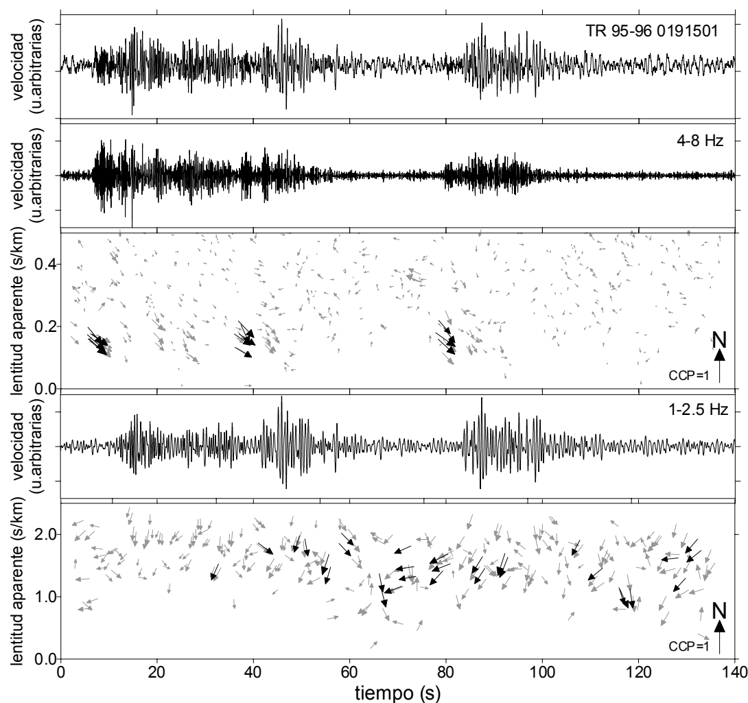
Figura 8.2. Resultados de la aplicación del método de la CCP a lo largo del tiempo a una señal registrada durante un tremor. La segunda parte de la señal es un evento híbrido. Obsérvese la presencia de dos paquetes de onda bien correlacionados durante el tremor, y la coincidencia en dirección y lentitud aparente con los valores obtenidos para el híbrido.
