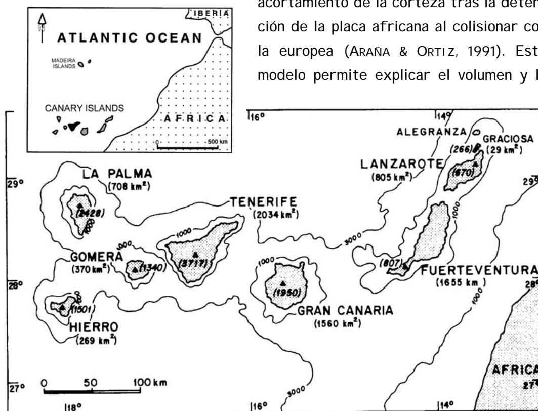
Figura 1.1. Situación del archipiélago de las islas Canarias (modificado de ARAÑA, 1995 y MARTÍ ET AL., 1995).
