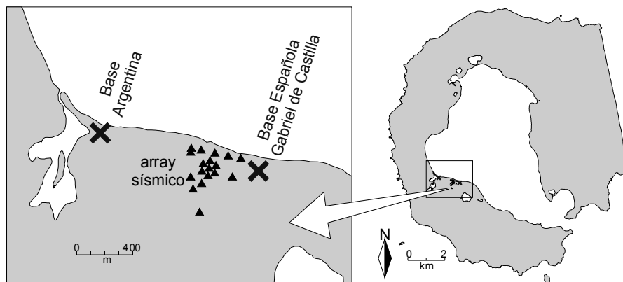
Figura 4.13. Situación del array sísmico de la isla Decepción, en las proximidades de la base Gabriel de Castilla.
