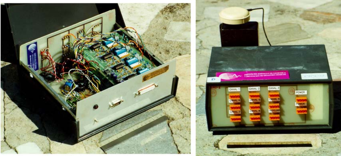
Figura 2.4. Última versión del sistema de adquisición de datos. Pueden verse los ocho conectores para los canales, la entrada de la alimentación, las puertas serie y paralelo y la antena del GPS.
