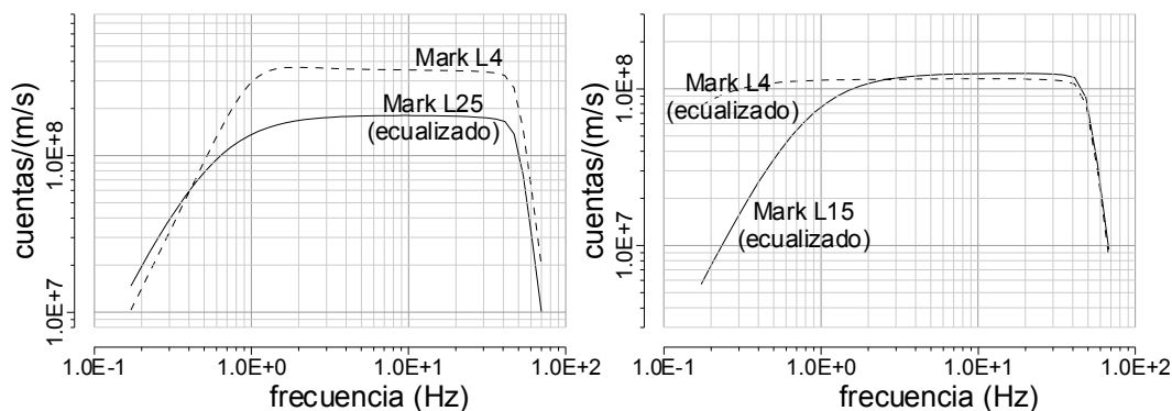
Figura 2.3. Curvas de respuesta de algunos de los instrumentos instalados.
