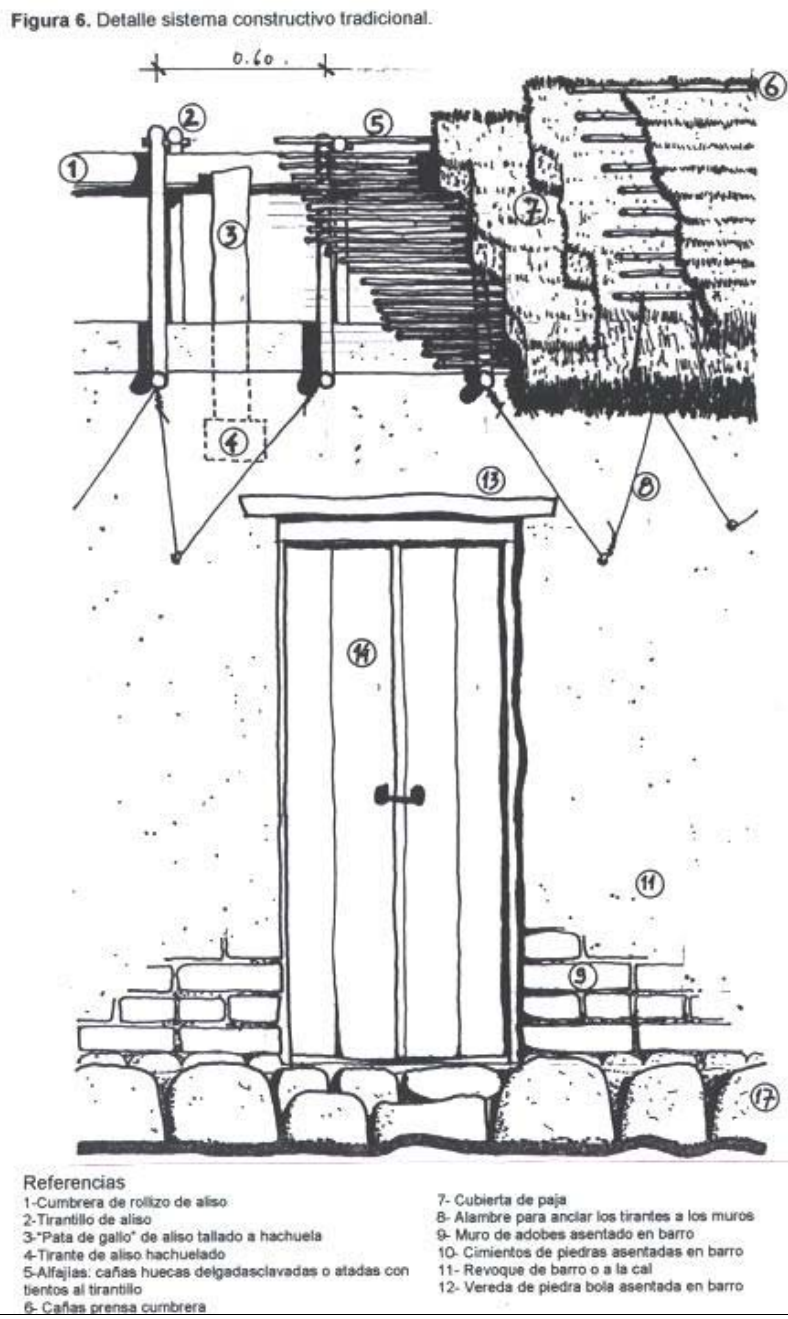
Figura 6. Detalle sistema constructivo tradicional.
