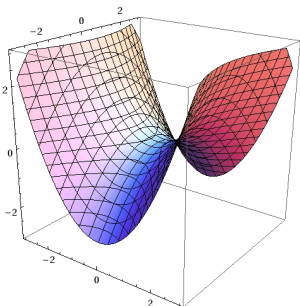
XI. paraboloide hiperbólico
