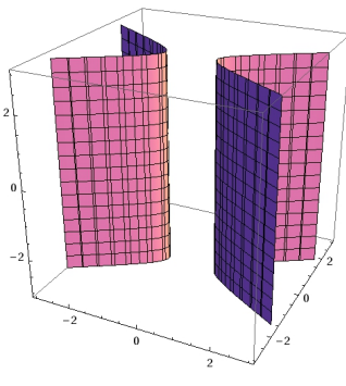
IX Cilindro hiperbólico
