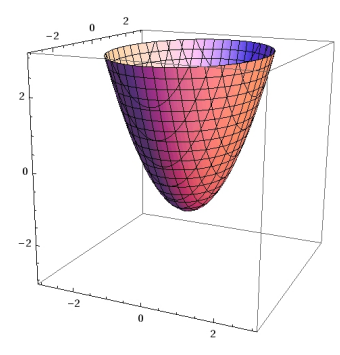
X. Paraboloide elíptico
