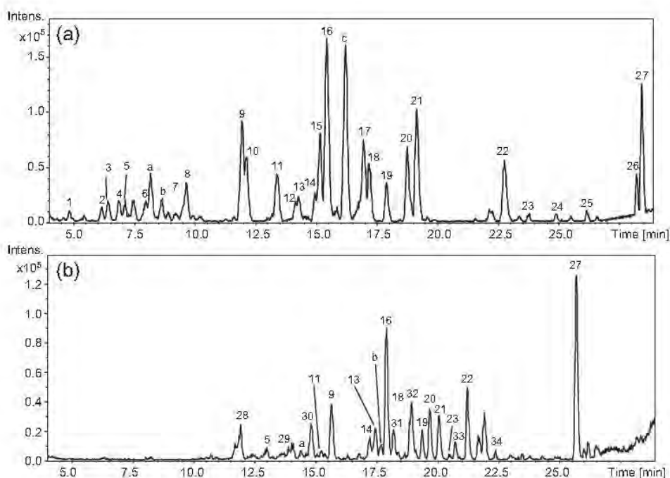
Figure 9.1. Perfil cromatográfico usando los programas de gradiente: (a) cromatograma para el programa de gradiente 1 en modo de ionización negativo; (b) cromatograma para el programa de gradiente 2 en modo de ionización positivo.
