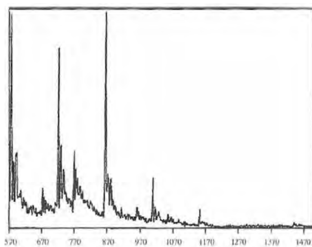
Figura 6.8. Perfil de PAC del extracto de arándano americano Fraccionado por ESI-MS 34 .
