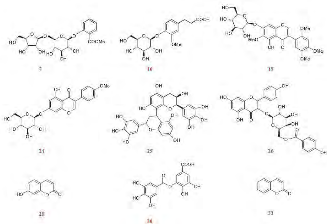
Figura 9.2. Estructura de los nuevos componentes identificados en el jarabe de arándano americano (7) cantosido A, (10) ácido dihidroferulico 4-O- \beta -D-glucuronido, (15) caviunina glucosido, (24) biochanina A-7-O-glucosido, (25) prodelfinidina B4, (26) kempferol 3-O- \beta -d-(6-p-hidroxibenzoil)-galactopiranosido, (28) 7-hidroxicumarina, (30) ácido digalico y (31) cumarina 48 .
