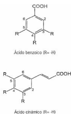
Figura 6.11. Estructuras de los ácidos benzoico y cinámico ( R = -H ). 34 .
