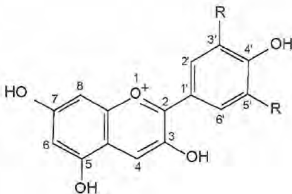
Figura 6.9. Estructura general de las antocianidinas (aglicones de los antocianósidos o antocianinas).
